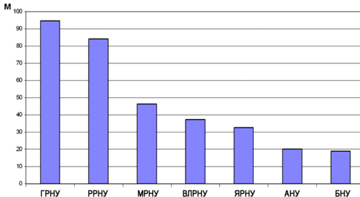
Рисунок 8-4.2 Ранжирование ОПО по удельным материальным потерям нефти
