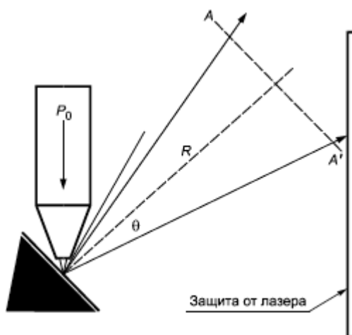
Рисунок В.2 - Расчет зеркального отражения
