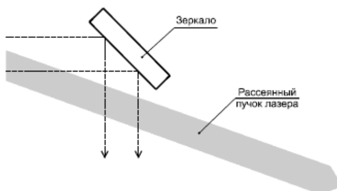
Рисунок В.4b - Отклонение пучка от зеркала во время процедуры регулировки
