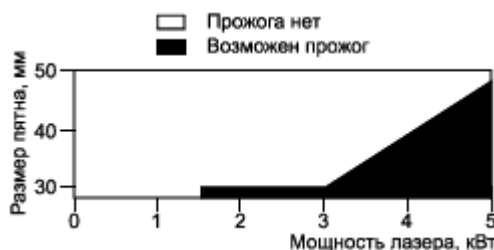
Рисунок F.1 - Стойкость к разрушению листа оцинкованной стали толщиной 1 мм от 10 с экспозиции расфокусированного пучка во время экспериментов с использованием непрерывного лазера на углекислом газе
