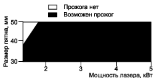
Рисунок F.10 - Стойкость к разрушению листа нержавеющей стали толщиной 1 мм от 100 с экспозиции расфокусированного пучка во время экспериментов с использованием непрерывного лазера на углекислом газе
