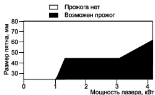
Рисунок F.20 - Стойкость к разрушению листа алюминия толщиной 2 мм от 100 с экспозиции
