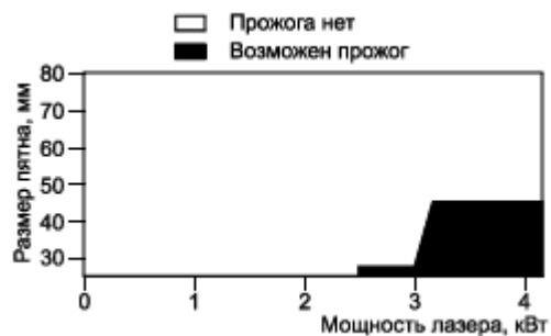
Рисунок F. 19 - Стойкость к разрушению листа алюминия толщиной 2 мм от 10 с экспозиции расфокусированного пучка во время экспериментов с использованием непрерывного лазера на иттрий-алюминиевом гранате с неодимом
