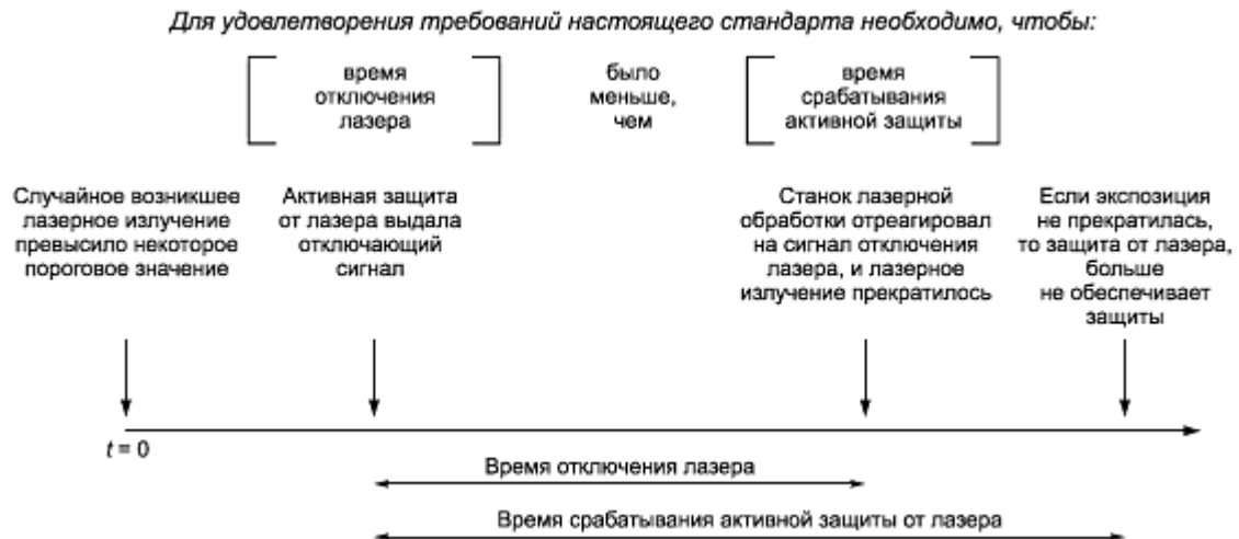
Рисунок С.2 - Пример параметров активной защиты от лазера
