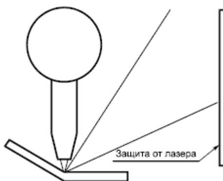
Рисунок В.3б - Изгиб заготовки или неправильное ее крепление
