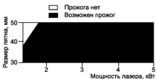
Рисунок F.11 - Стойкость к разрушению листа поликарбоната толщиной 6 мм от 10 с экспозиции расфокусированного пучка во время экспериментов с использованием непрерывного лазера на углекислом газе
