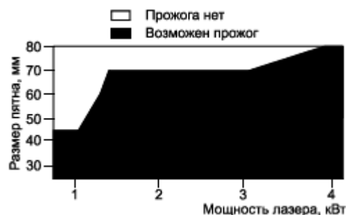
Рисунок F.14 - Стойкость к разрушению листа оцинкованной стали толщиной 1 мм от 100 с экспозиции расфокусированного пучка во время экспериментов с использованием непрерывного лазера на иттрий-алюминиевом гранате с неодимом
