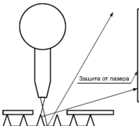
Рисунок В.3с - Отсутствие заготовки
