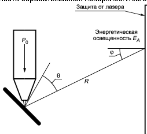
Рисунок В.1 - Расчет диффузного отражения
