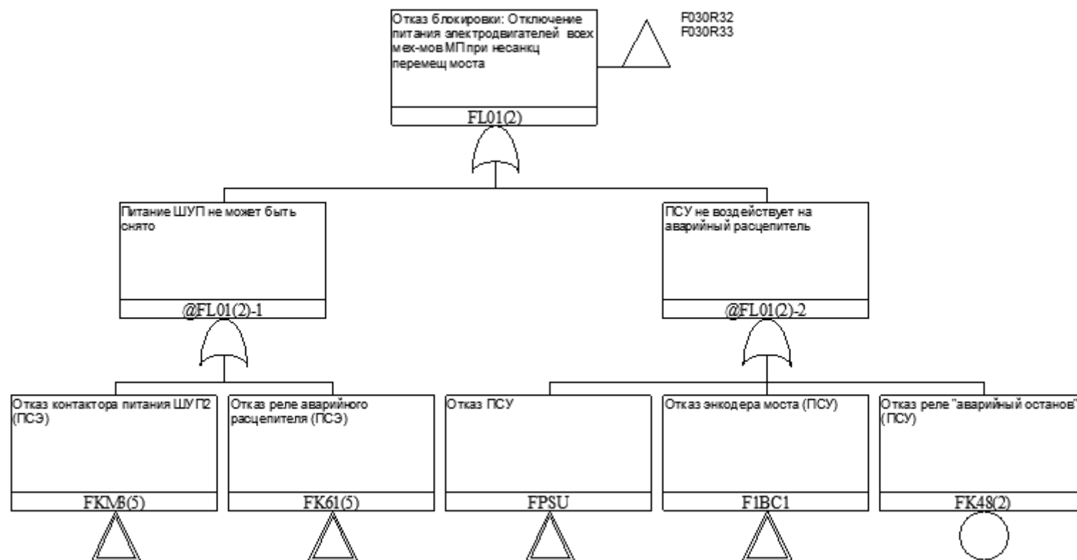
Рис.5. Дерево отказов "Отказ блокировки: Отключение питания электродвигателей всех механизмов МП при несанкционированном перемещении моста" (построено на основе анализа защит и блокировок МП)
