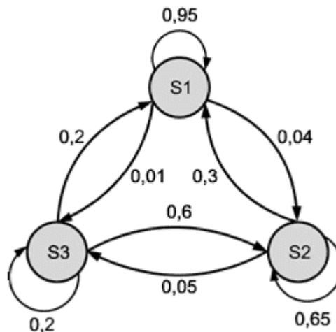
Рисунок В.9 - Пример диаграммы Маркова для системы
