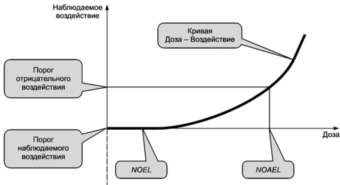
Рисунок В.1 - Кривая Доза - Воздействие
