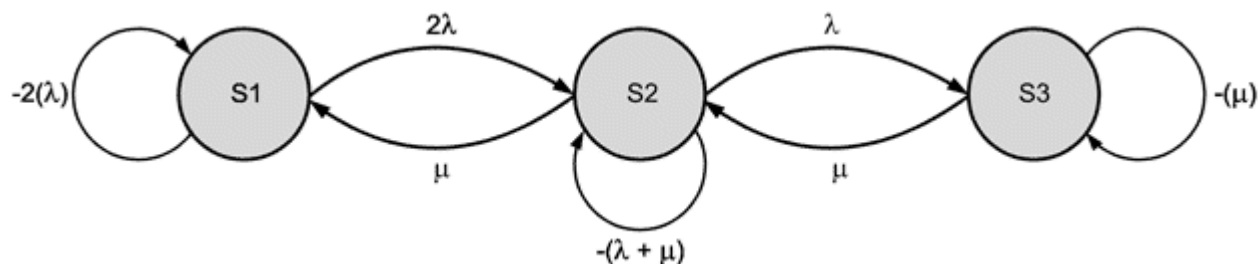
Рисунок В.10 - Пример диаграммы состояний перехода
