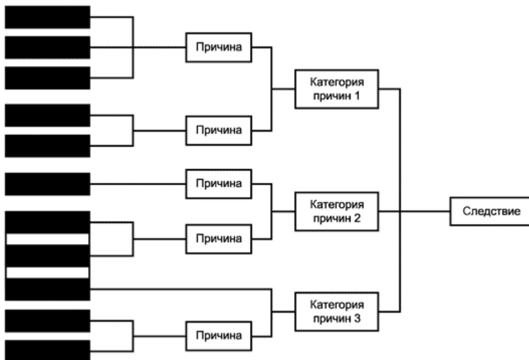
Рисунок В.6 - Пример представления причинно-следственного анализа в виде древовидной структуры В.17.5 Выходные данные
