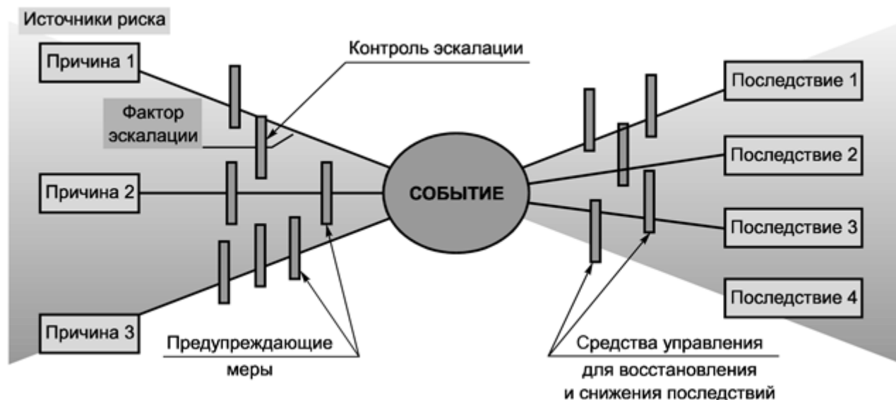
Рисунок В.8 - Пример диаграммы "галстук-бабочка" для нежелательных последствий В.21.6 Преимущества и недостатки
