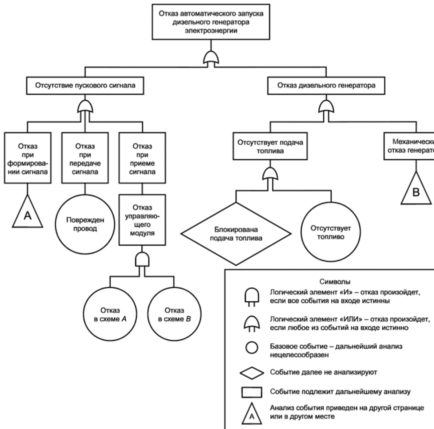
Рисунок В.2 - Пример метода FTA
