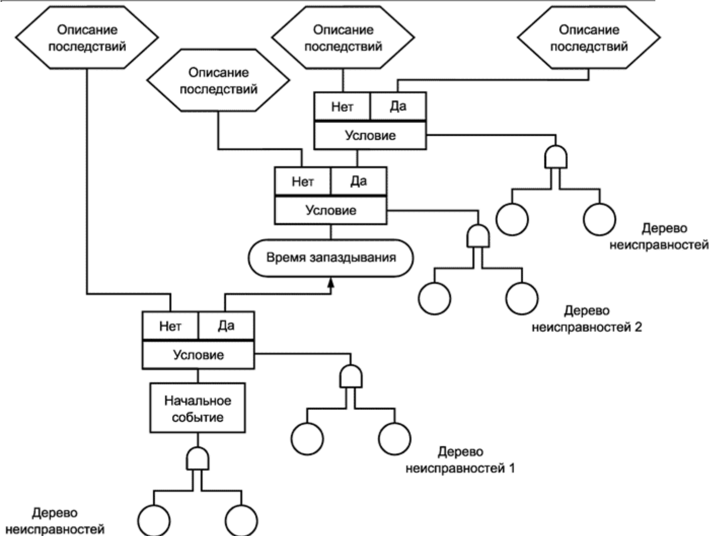
Рисунок В.4 - Пример анализа причин и последствий
