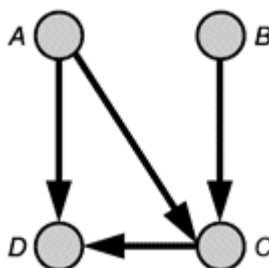
Рисунок В.11 - Пример сети Байеса
