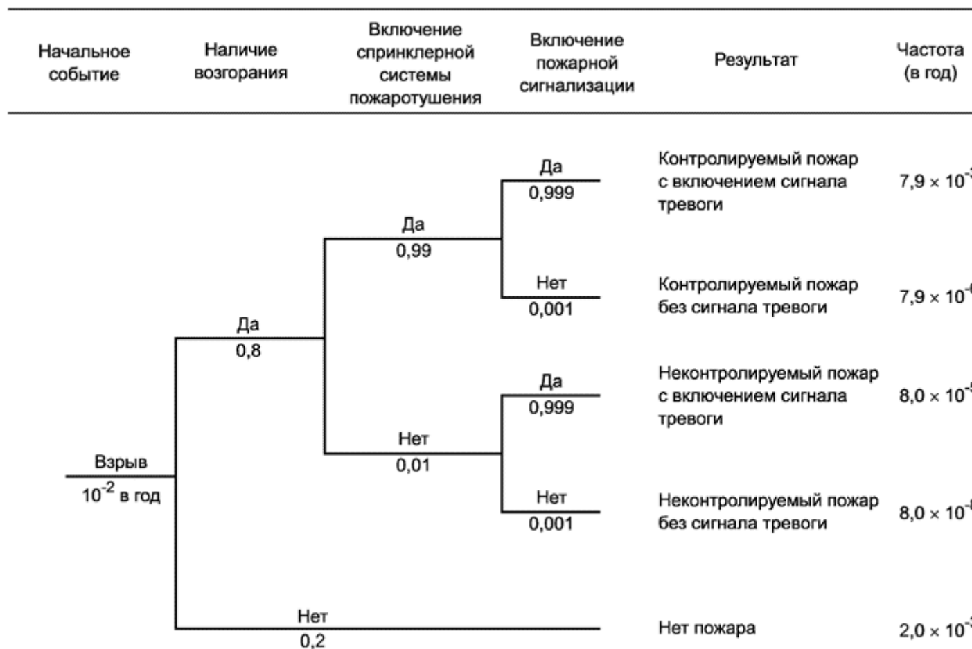
Рисунок В.3 - Пример дерева событий
