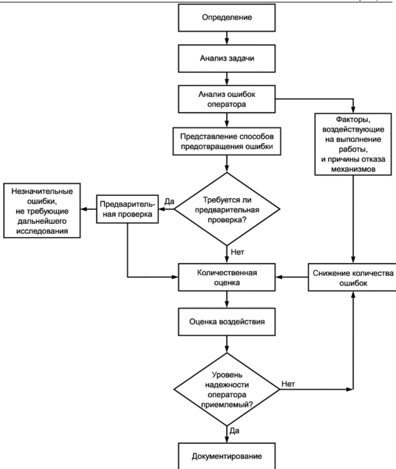
Рисунок В.7 - Пример анализа влияния человеческого фактора В.21 Анализ "галстук-бабочка"
