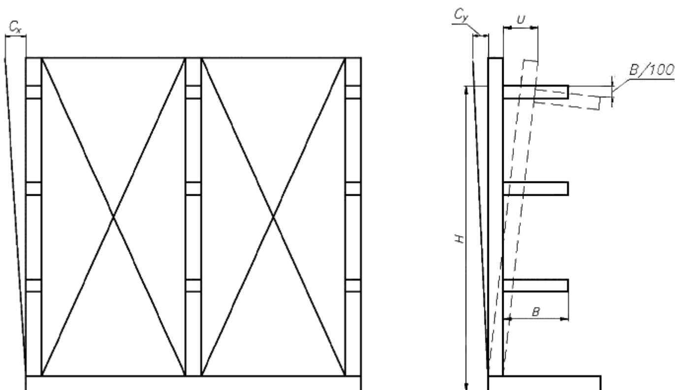
Рисунок 13 - Прогиб элементов консольных стеллажей Параметры отклонения стоек от вертикальной плоскости:
