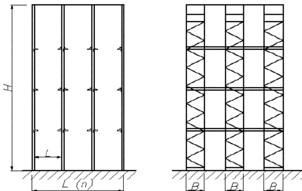
Рисунок 1 - Общий вид фронтального стеллажа Набивной (глубинный) стеллаж
