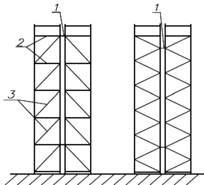
1 - межрамная связь; 2, 3 - элементы раскосной системы.
