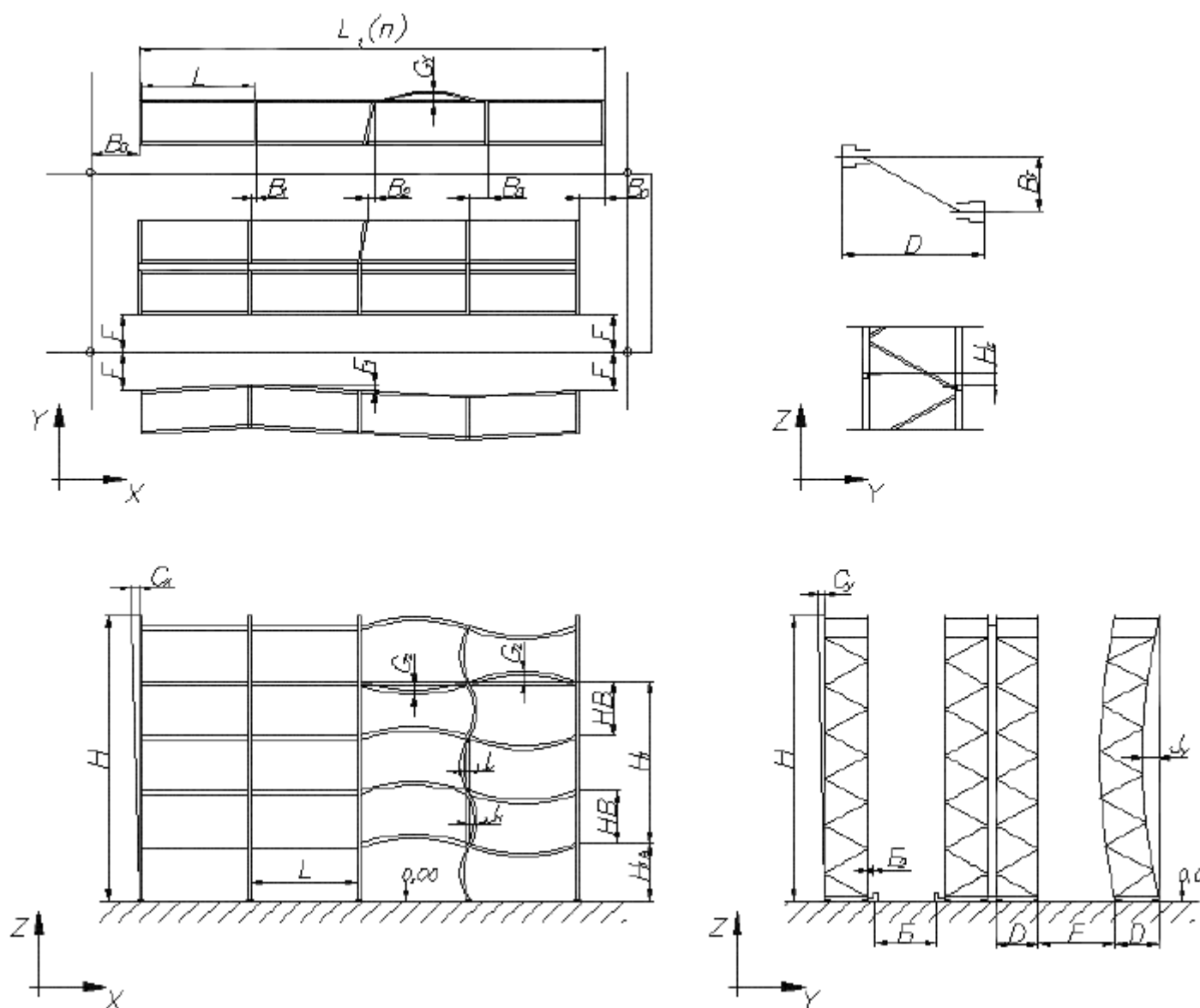
Рисунок 7 - Параметры, подлежащие контролю в ненагруженном состоянии системы
