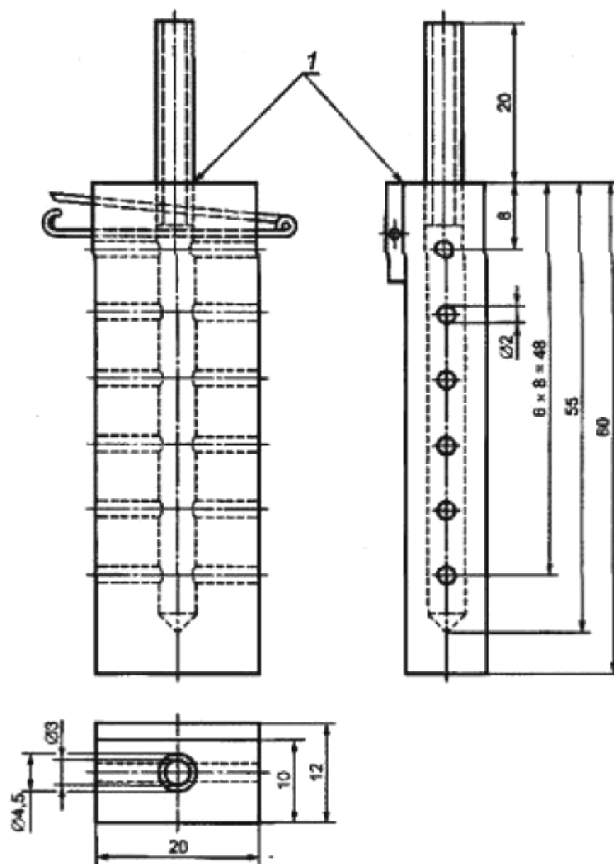
Рисунок А.3 - Пробоотборник
