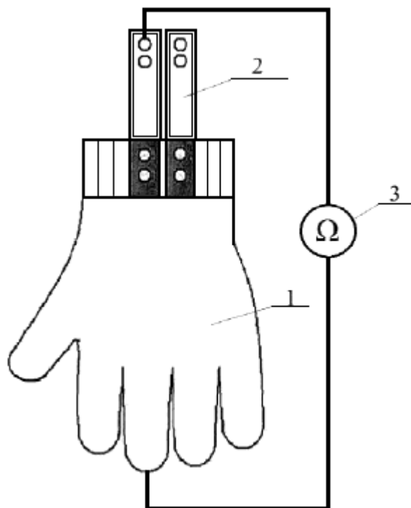
1 - защитная перчатка; 2 - контактный вывод; 3 - омметр
