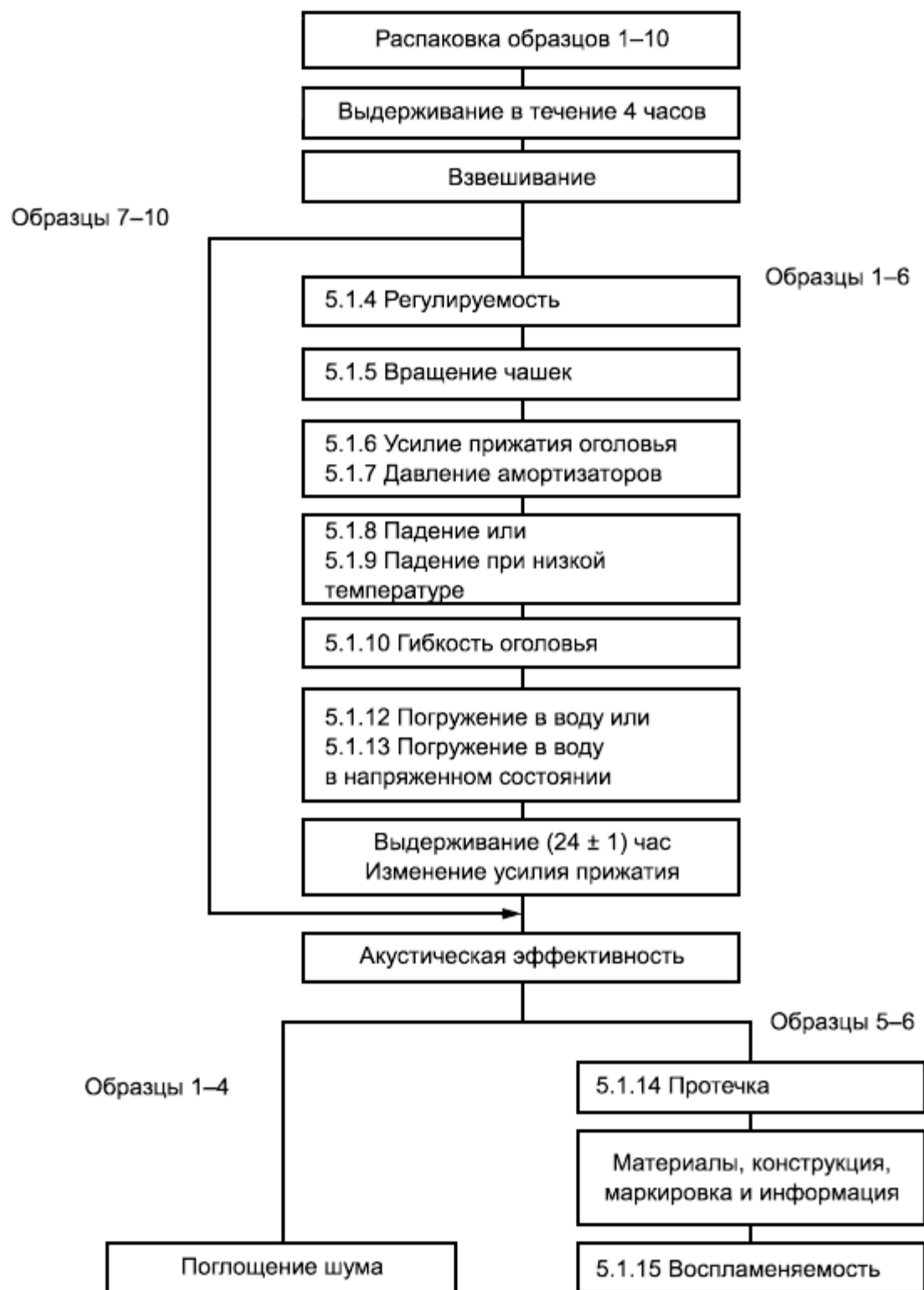
Рисунок В.1 - Блок-схема испытаний наушников с оголовьем
