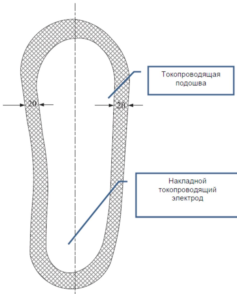
Рисунок 2 - Схема наложения накладного токопроводящего электрода
