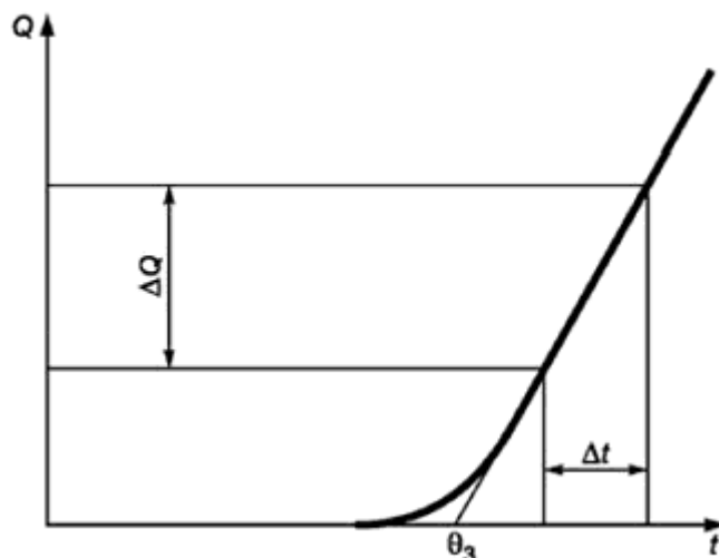
Рисунок 5 - Кривая изменения количества проникшей жидкости Q во времени t 5.2.2 Сорбирующая среда
