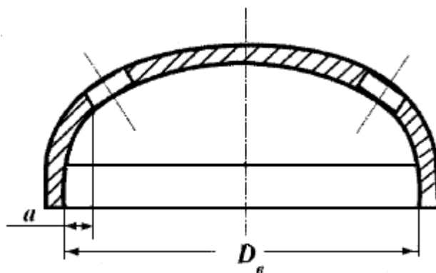
Рис.4. Расположение отверстий в днище
