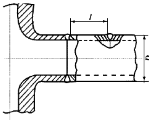
Рис.12. Расположение сварных соединений трубопровода с патрубком
