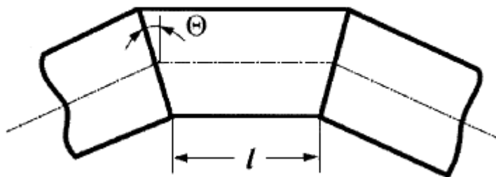
Рис.6. Схема секторного отвода
