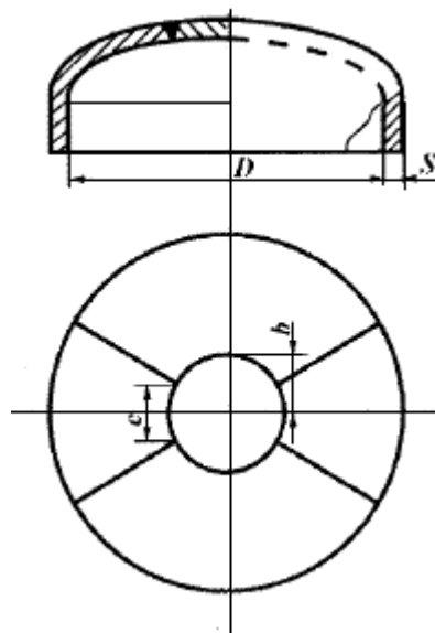
Рис.9. Расположение радиальных и круговых швов
