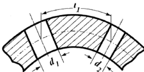
Рис.3. Расположение отверстий на криволинейной поверхности
