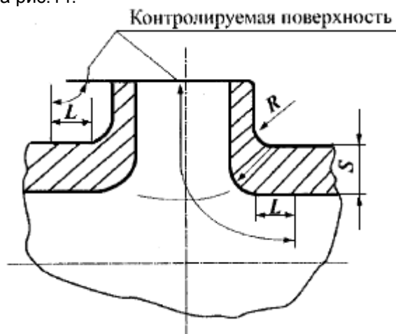
Рис.14. Схема высадки горловины, L \geq 30 мм
