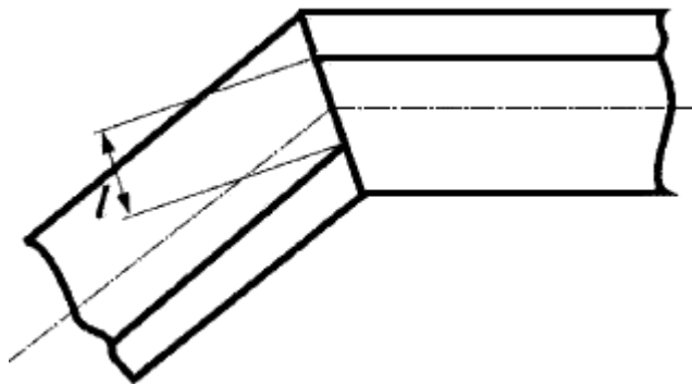
Рис.7. Расположение сварных соединений в секторных отводах
