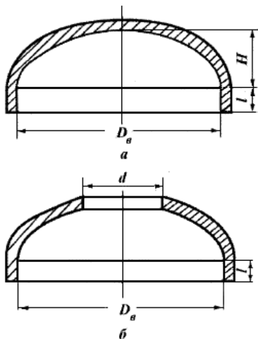
Рис.1. Эллиптическое днище: а - без отверстия; б - с отверстием
