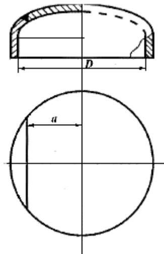
Рис.8. Расположение хордовых швов
