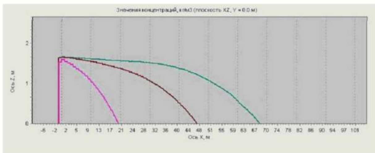
Рисунок 9-10. Зоны достижения концентрацией ВКПР, НКПР и 0,5 НКПР в вертикальной плоскости, проходящей через ось выброса, при выбросе пропана (пример 4)
