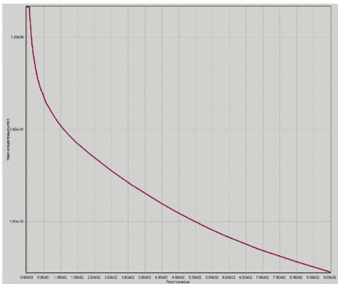
Рисунок 9-1. Максимальная приземная концентрация на оси облака (по направлению ветра) при выбросе хлорметана (пример 1)
