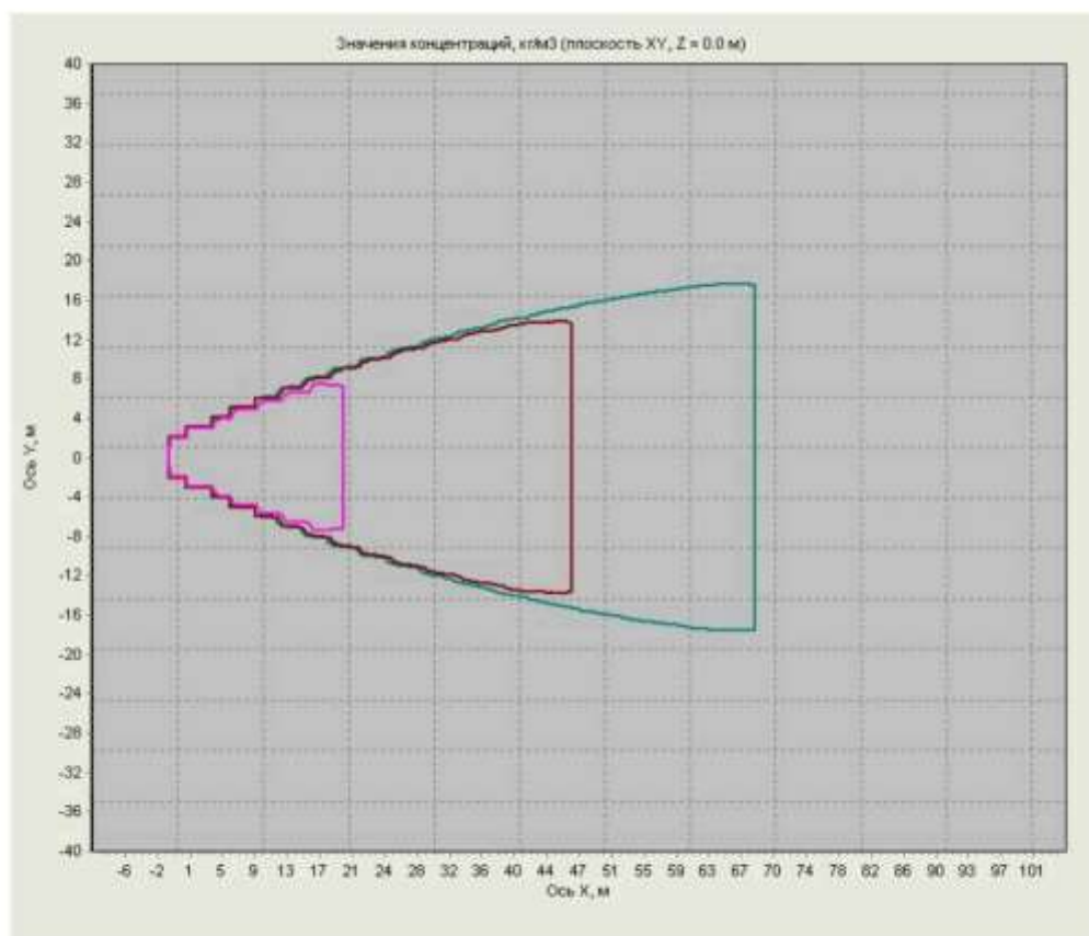
Рисунок 9-9. Зоны достижения концентрацией ВКПР, НКПР и 0,5 НКПР на поверхности земли при выбросе пропана (пример 4)
