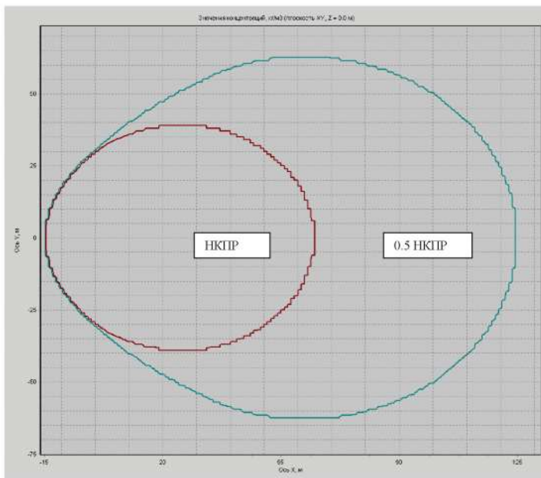
Рисунок 9-2. Сечение зоны, ограниченной НКПР и 0,5 НКПР плоскостью, z=0 (в направлении по ветру) при выбросе хлорметана (пример 1)
