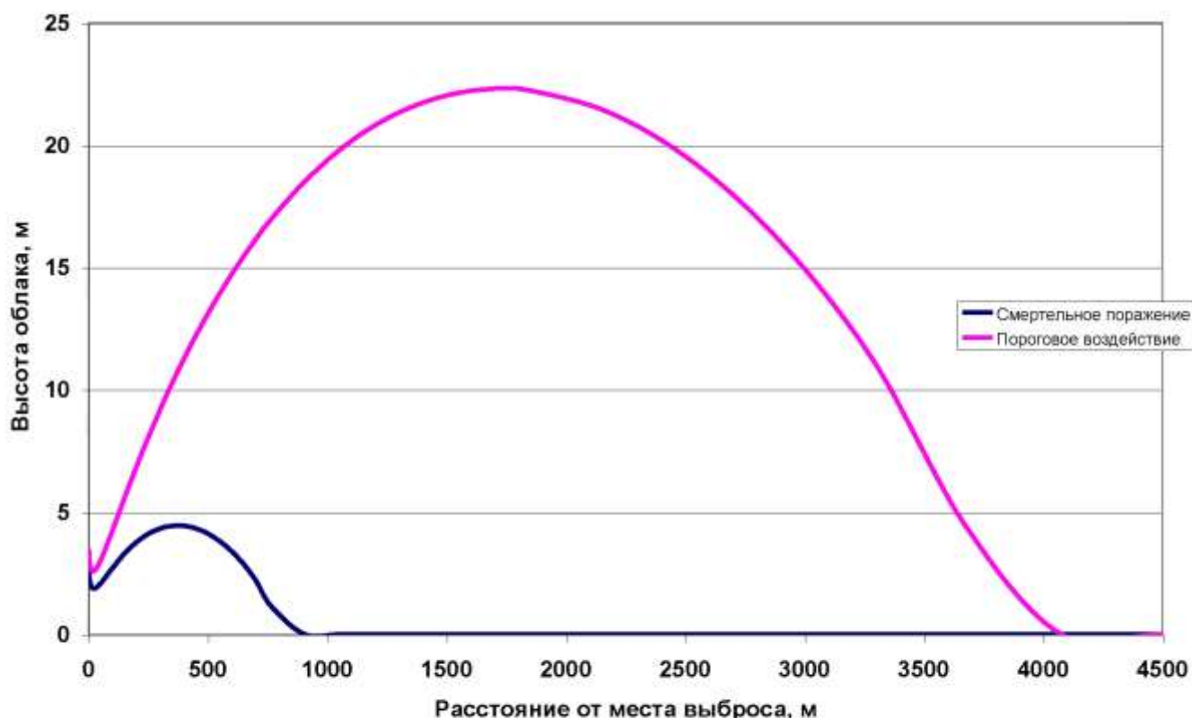
Рисунок 9-5. Размеры зоны смертельного поражения в плоскости y=0 (вертикальное сечение через ось выброса) при выбросе хлорциана (пример 2)
