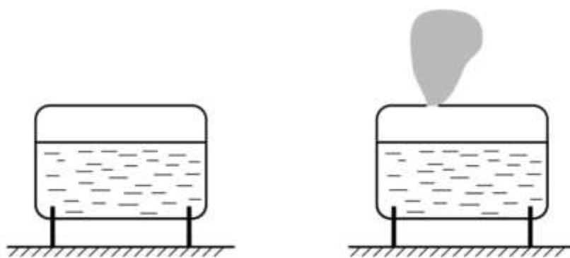
Рисунок 4-4. Разгерметизация емкости с жидкой фазой выше уровня жидкости (сценарий 4)
