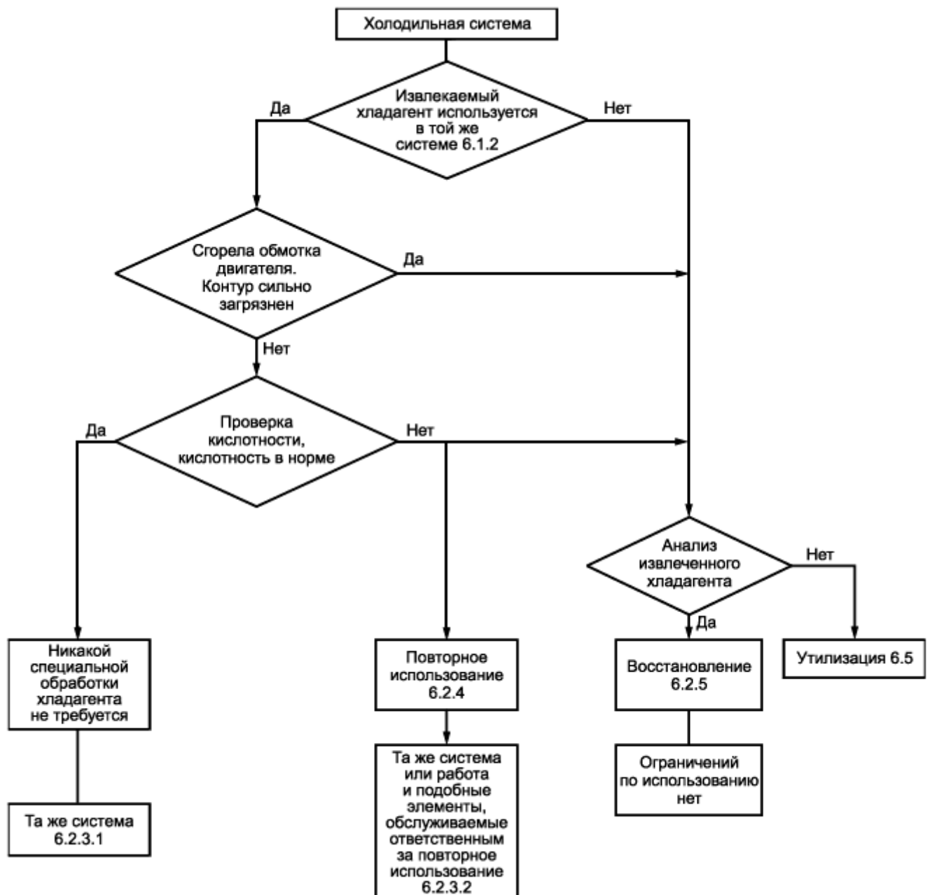
Рисунок 2 - Блок-схема операций, выполняемых при извлечении хладагента 6.2.3.2 Использование в аналогичной системе
