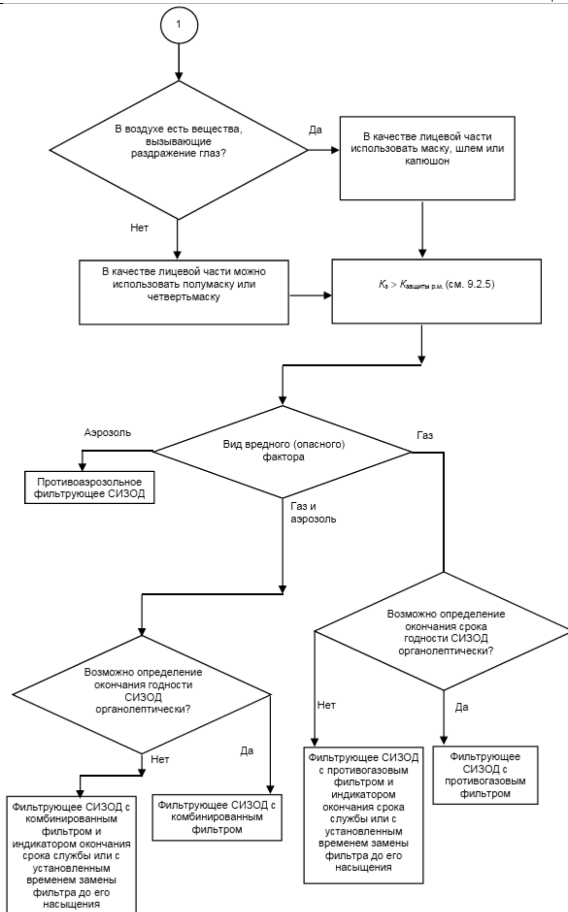
Рисунок В.1 - Алгоритм выбора СИЗОД
