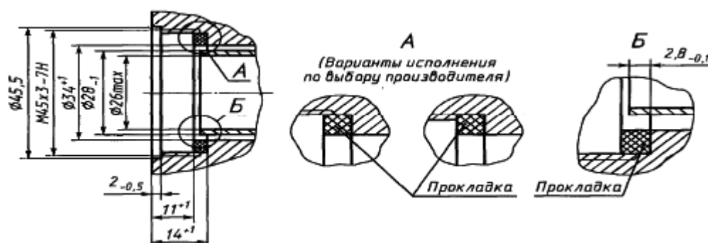
Рисунок Б.4 - Резьбовое соединение с внутренней резьбой для систем с двумя каналами подачи воздуха PIB
