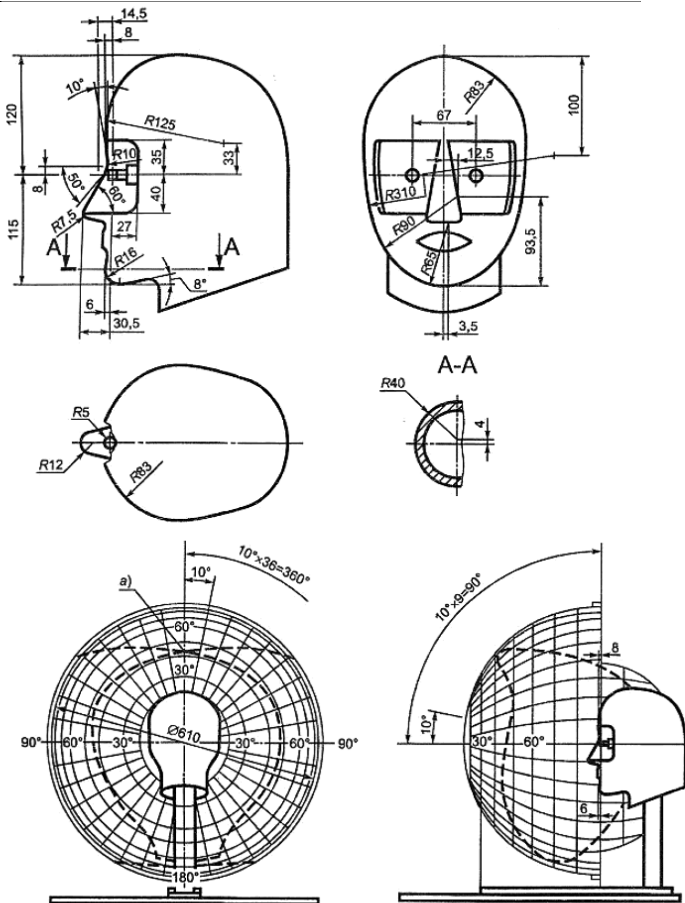
Рисунок 14 - Апертометр
