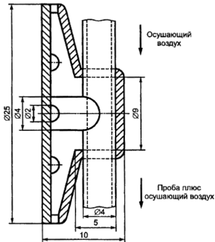
Рисунок 11 - Пробоотборник
