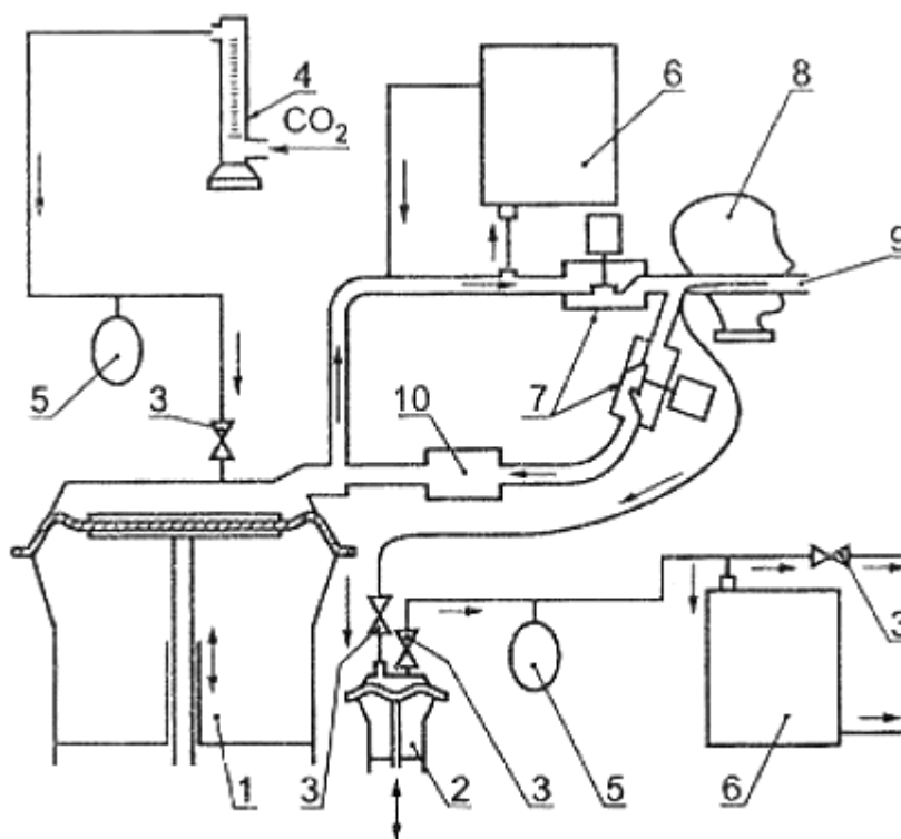
Рисунок 6 - Шеффилдская голова-манекен для испытания по определению содержания диоксида углерода во вдыхаемом воздухе и сопротивления постоянному воздушному потоку
