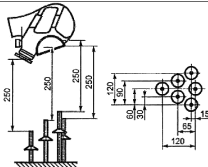
Рисунок 2 - Схема установки, состоящей из шести пропановых горелок
