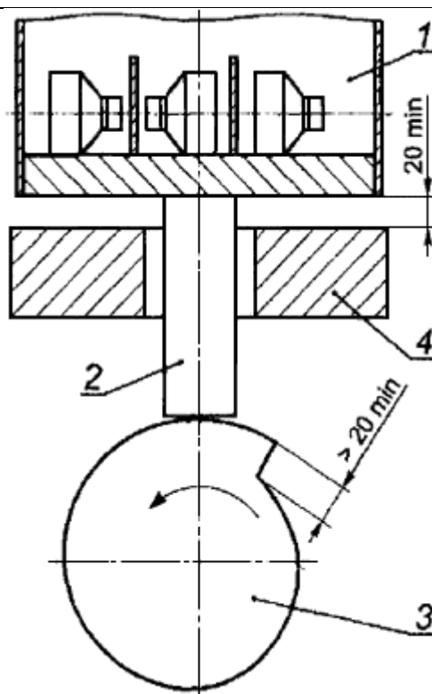
1 - стальная коробка; 2 - поршень; 3 - кулачок; 4 - стальная пластина
