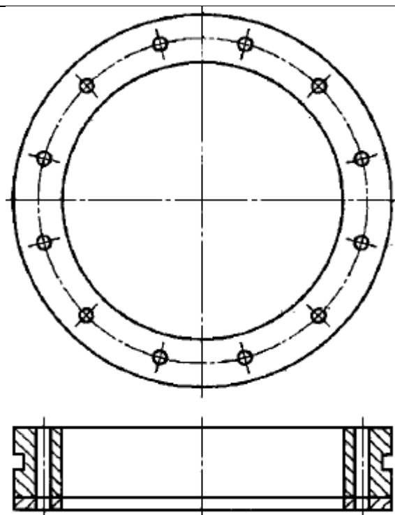
Рисунок А.1 - Скользящее кольцо
