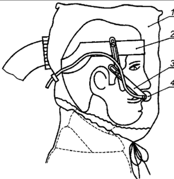
1 - испытуемый капюшон; 2 - оголовье; 3 - регулируемый пластмассовый кронштейн; 4 - проботборник
