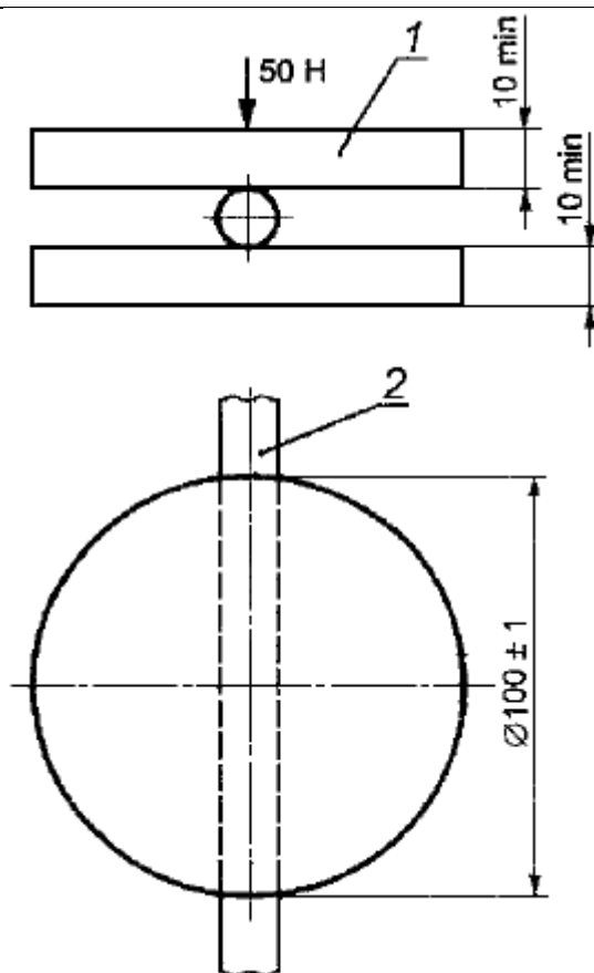
1 - подвижная пластина; 2 - дыхательный шланг
