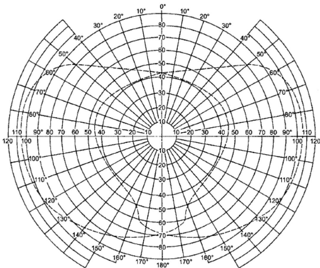
Рисунок 5 - Диаграмма апертометра
