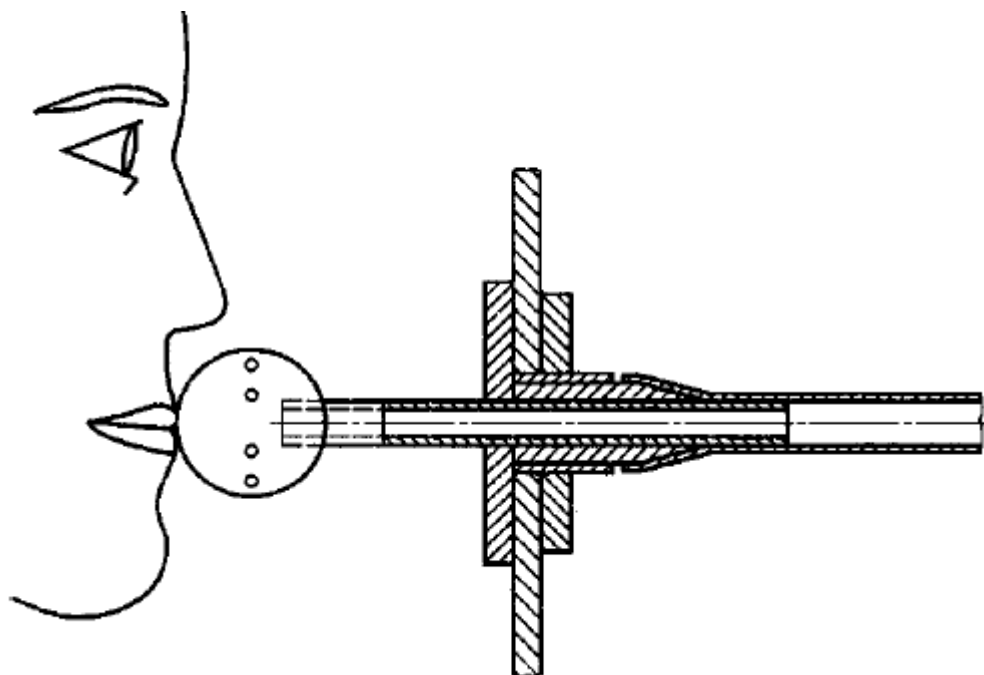
Рисунок 1 - Шариковый пробоотборник в устройстве с твердым смотровым стеклом
