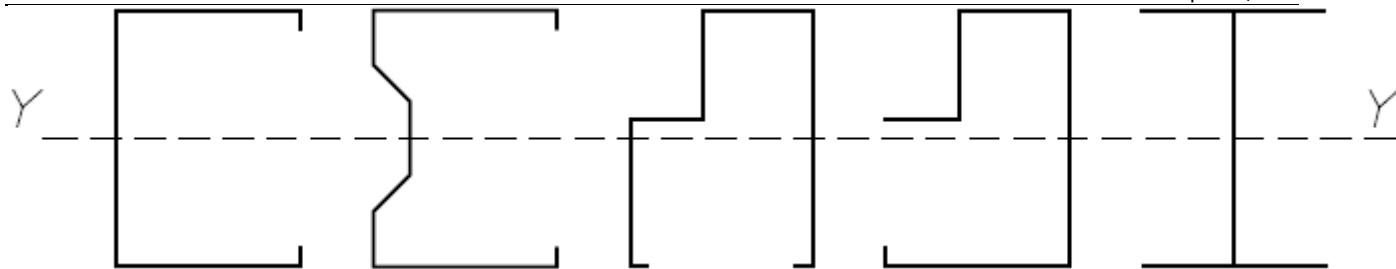
Рисунок 20 - Примеры балок, для которых вероятно потеря устойчивости плоской формы изгиба балок
