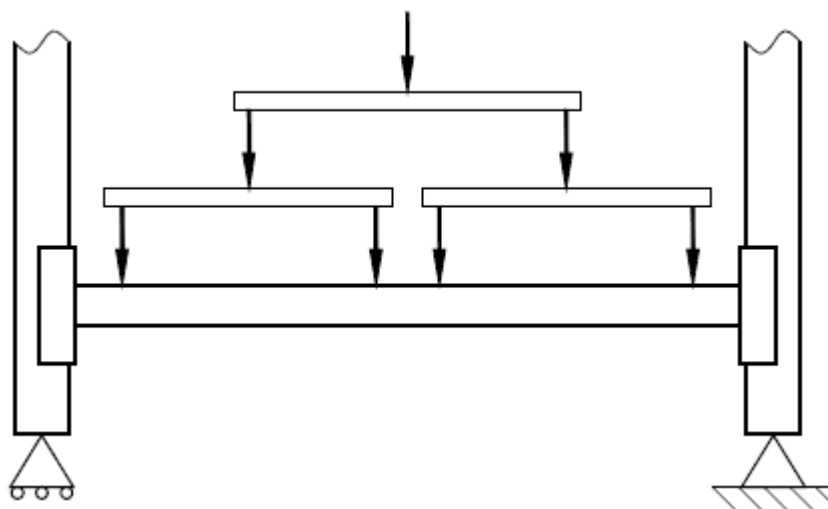
Рисунок А.16 - Пример моделирования нагрузки при испытаниях балок А.2.10.3 Порядок проведения испытаний
