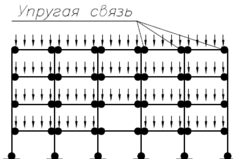
27a - Расчетная схема нагружения стеллажа без крестовых раскосов жесткости
