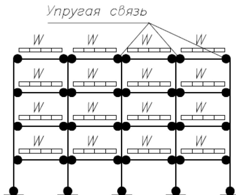
В.1а - Расчетная схема нагружения
