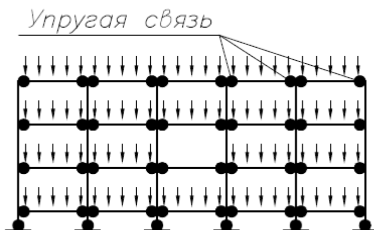
Рисунок 27с - Дополнительная схема нагружения при нахождении нижней балки возле уровня пола
