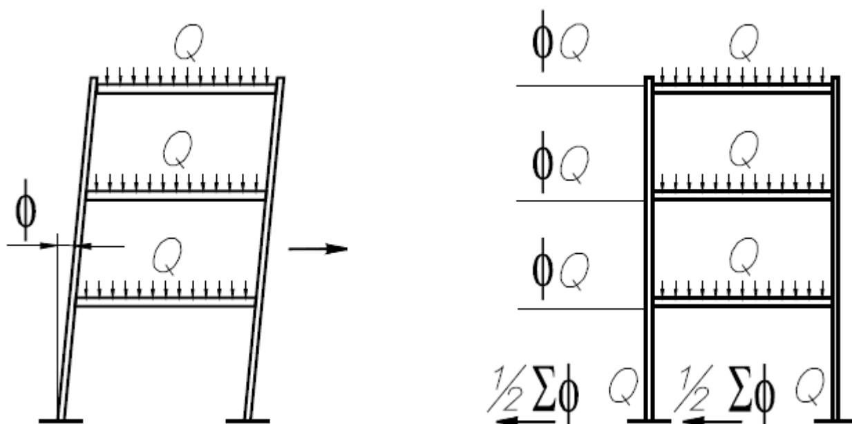
Рисунок 7 - Эквивалентные горизонтальные усилия
