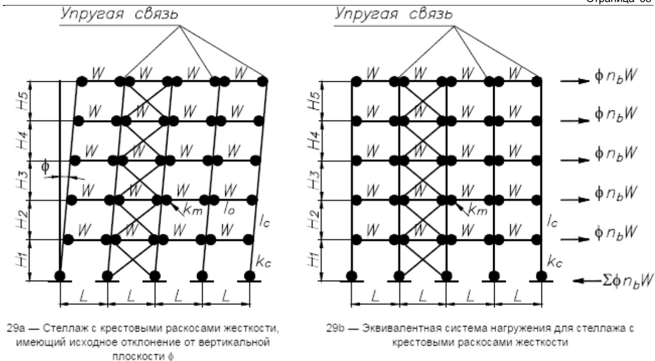
Рисунок 29 - Расчетная схема конструкции стеллажа с крестовыми раскосами жесткости для оценки устойчивости в X-направлении
