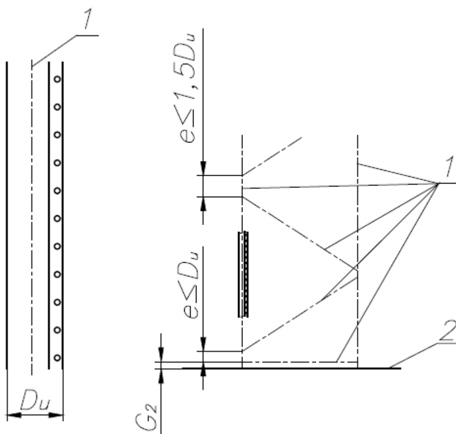
Рисунок 10а - Эксцентриситеты вертикального крестового раскоса жесткости
