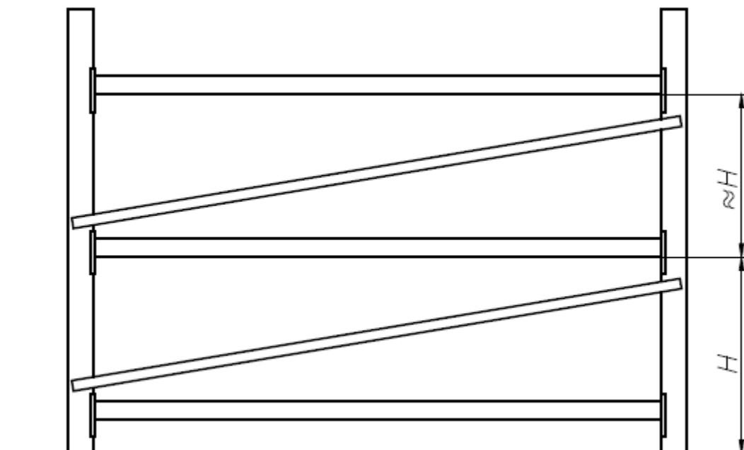
Рисунок 22b, вариант 2: Высота нижней балки над полом аналогична высоте между соседними балками
