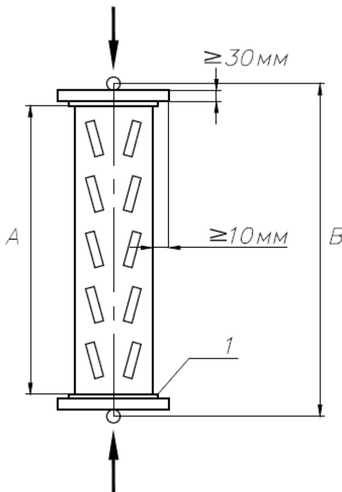
1 - опорные пластины; A - длина стойки; B - расчетная длина при продольном изгибе
