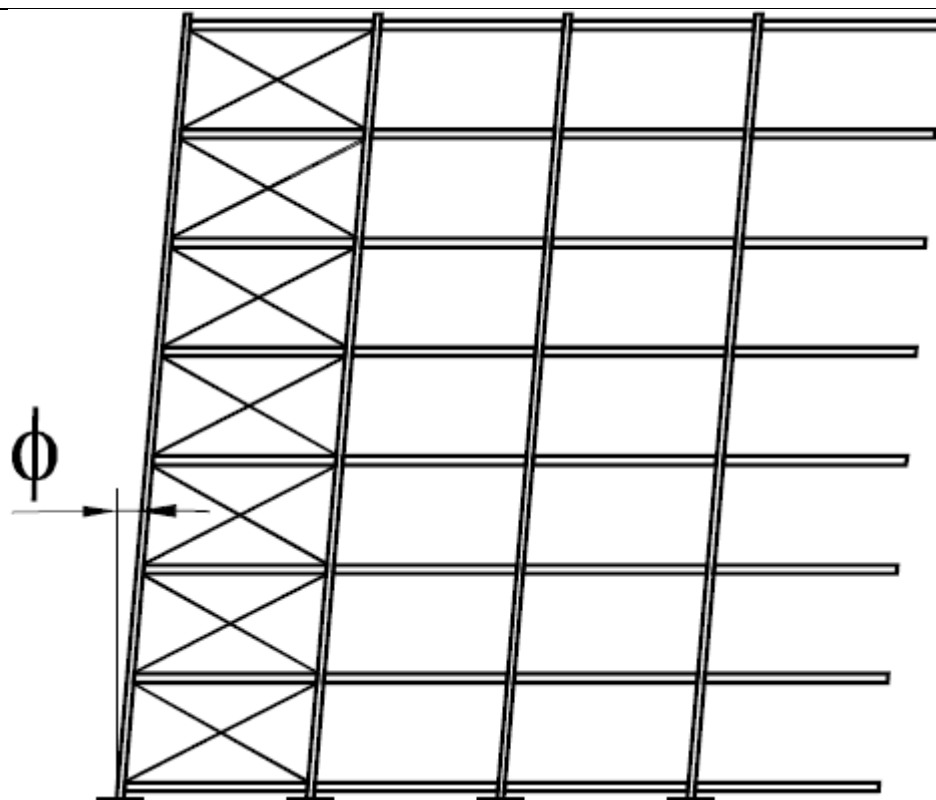
Рисунок 8 - Общие отклонения от вертикальной плоскости
