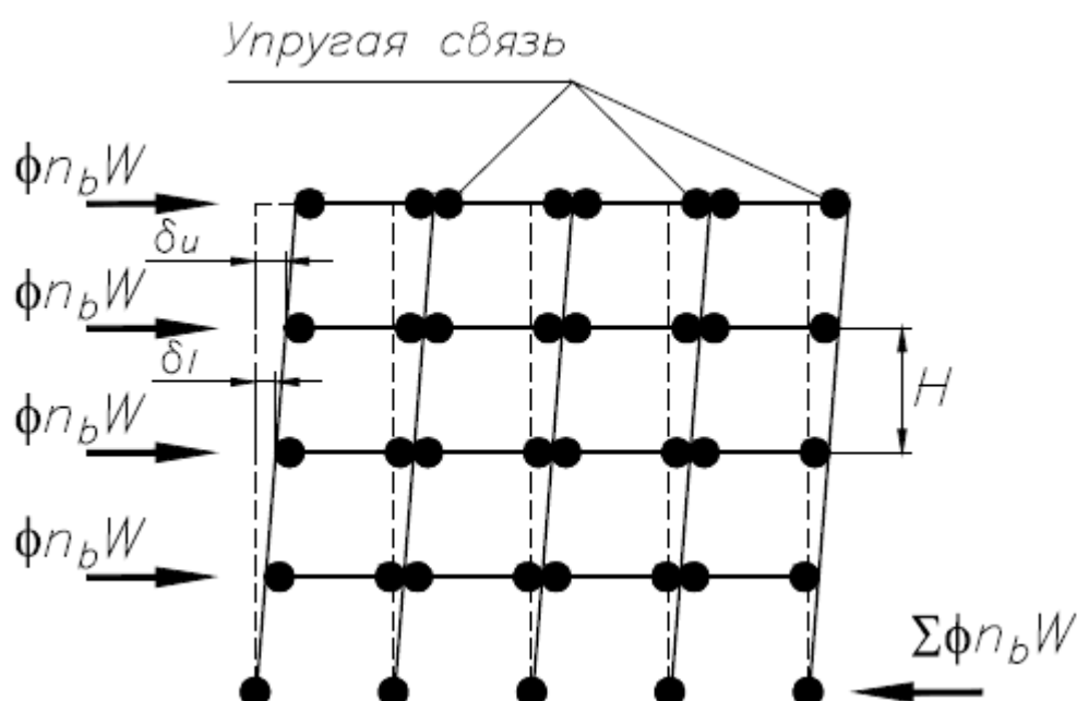
В.1b - Несовершенства от горизонтальных нагрузок и соответствующие отклонения
