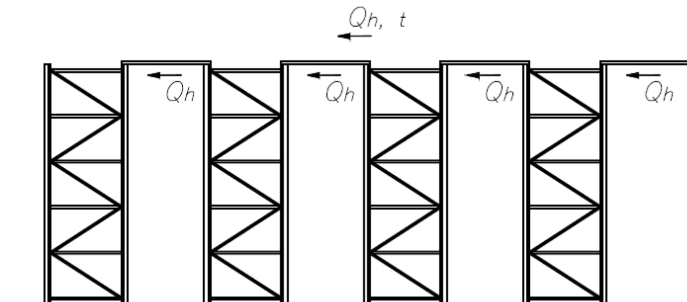
Рисунок 12 - Горизонтальные нагрузки от оборудования, опирающегося на конструкцию стеллажей Значения, указанные в таблице 1, не могут быть использованы в случае определения горизонтальной нагрузки Q_{h,t} как результата приложения односторонней несимметричной нагрузки к рельсу крана.
