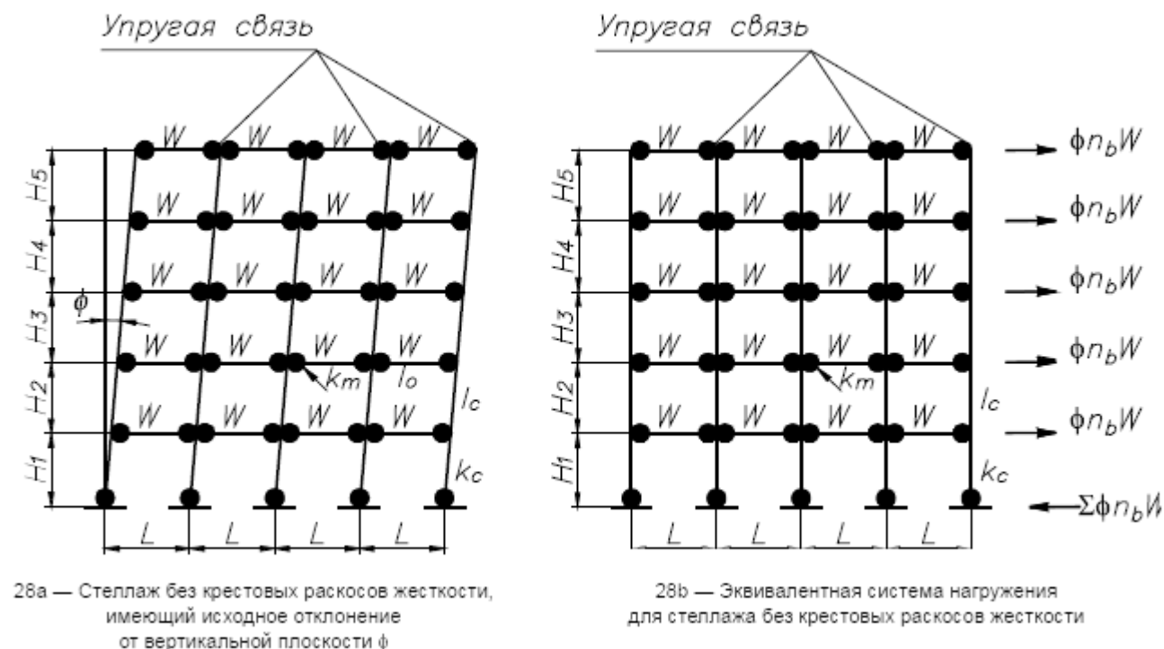
Рисунок 28 - Расчетная схема конструкции стеллажа без крестовых раскосов жесткости для оценки устойчивости в X-направлении
