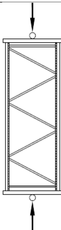
Рисунок А.4 - Порядок альтернативного проведения испытаний стоек на сжатие А.2.3.3 Метод проведения испытаний
