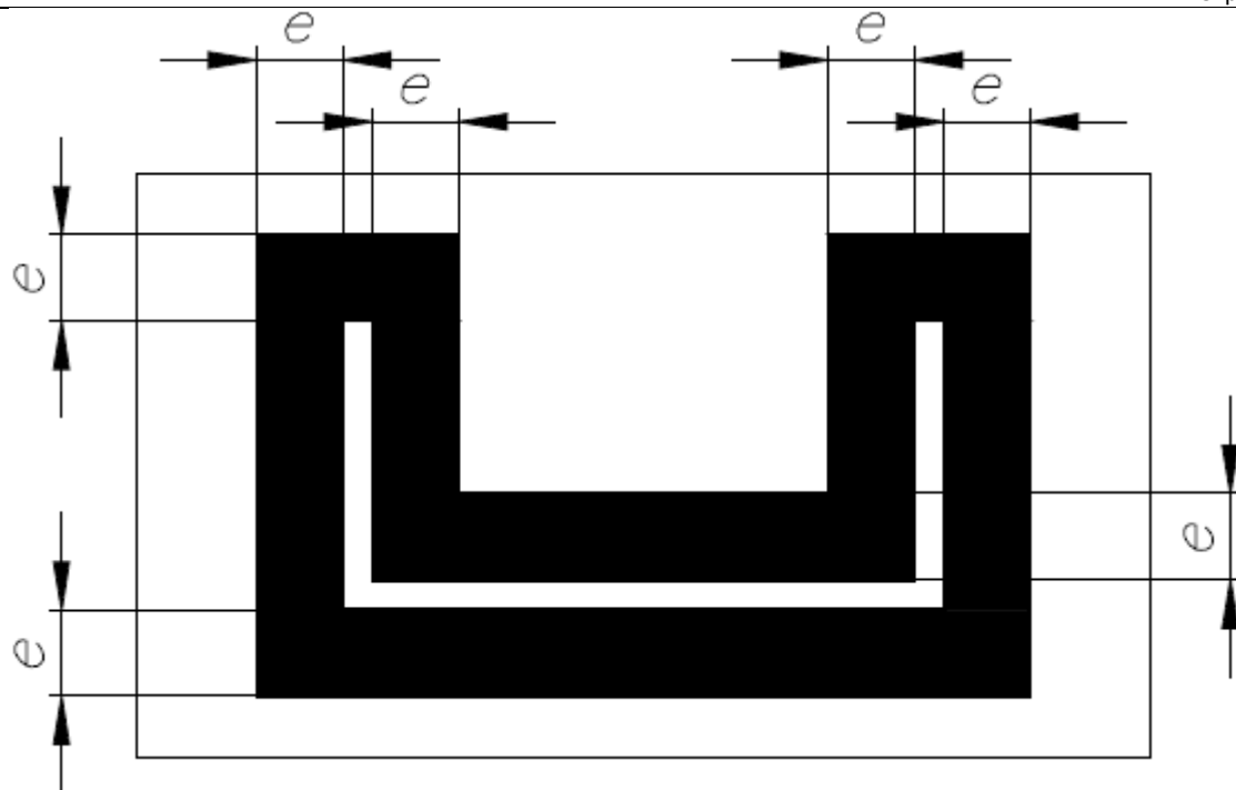
Рисунок 26 - Эффективная площадь для расчета подпятника
