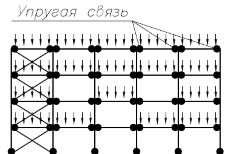
27b - Расчетная схема нагружения стеллажа с крестовыми раскосами жесткости
