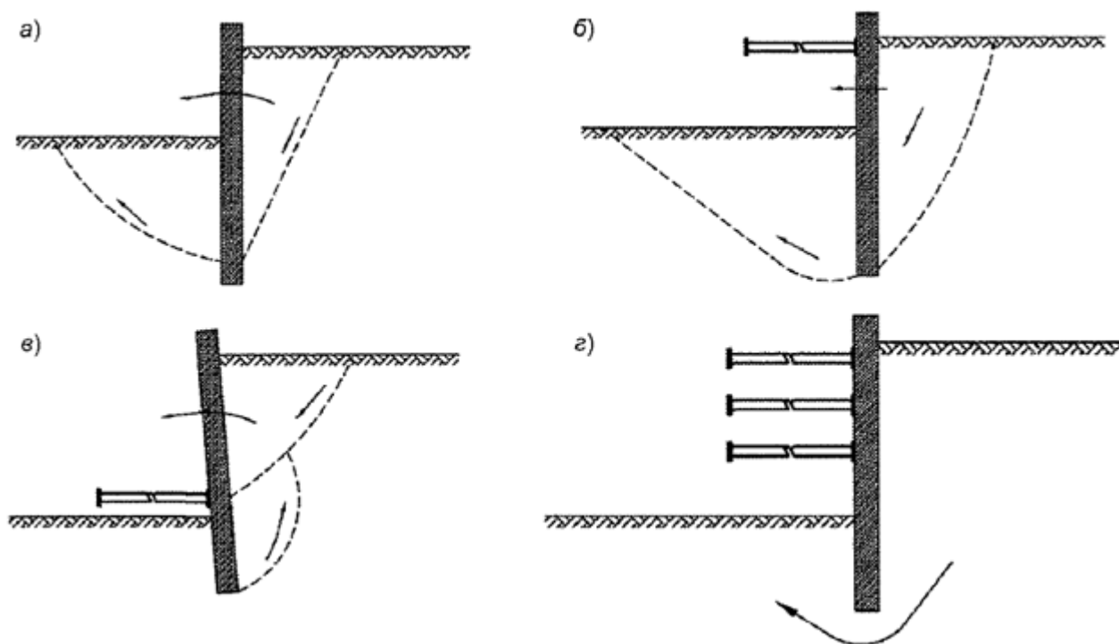
Рисунок 11.2 - Схемы разрушения при недостаточной заделке ограждения котлована
