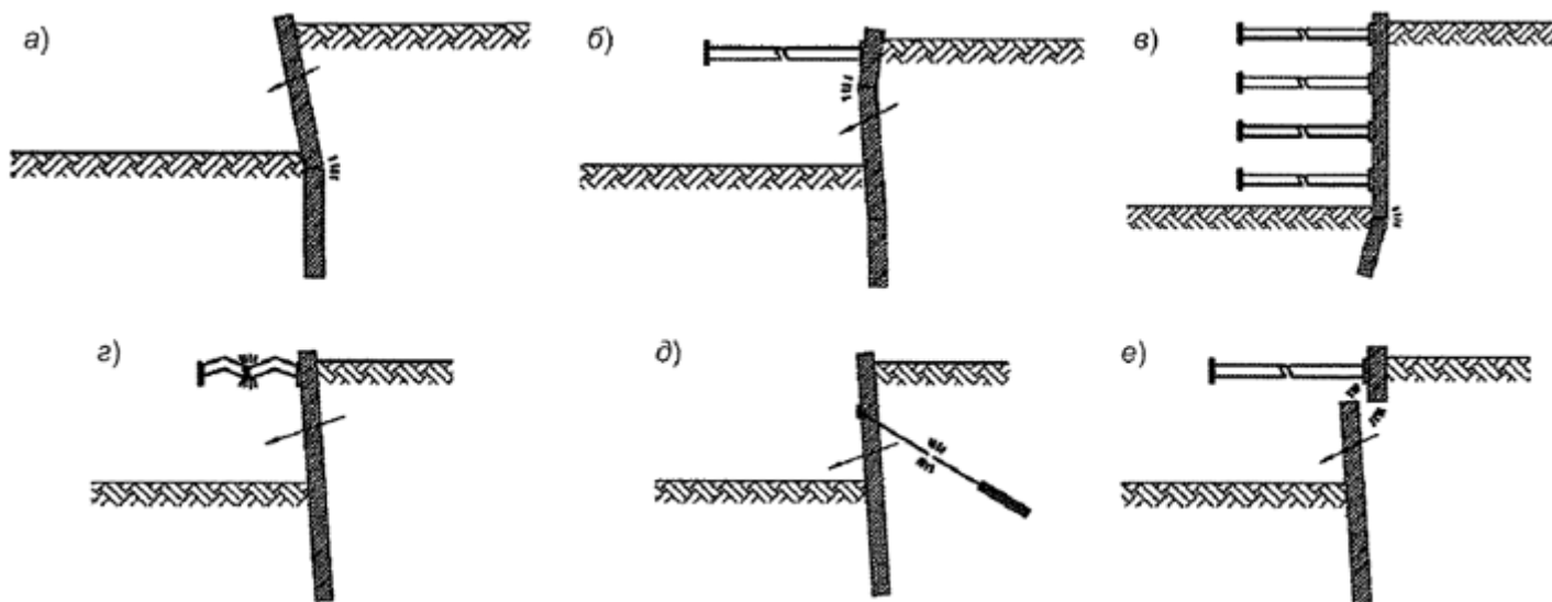
Рисунок 11.3 - Проектные ситуации, соответствующие разрушению конструктивных элементов
