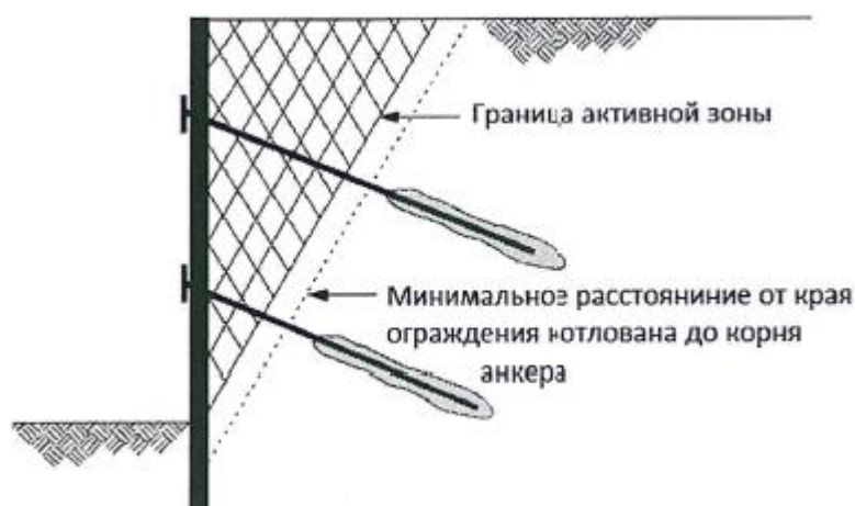
Рисунок 12.1 - Рекомендуемое расположение корней анкеров по отношению к активной зоне
