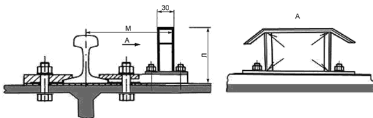
Рисунок В.3 - Типовая конструкция отключающей линейки
