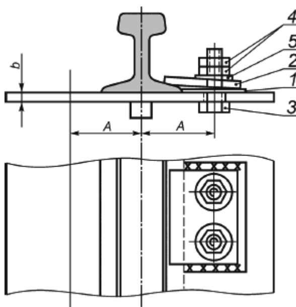
Рисунок Б.1 - Узел крепления по ГОСТ 24741 кранового рельса КР к стальной подкрановой балке Таблица Б.1 - Элементы узла крепления по ГОСТ 24741 кранового рельса КР к стальной подкрановой балке
