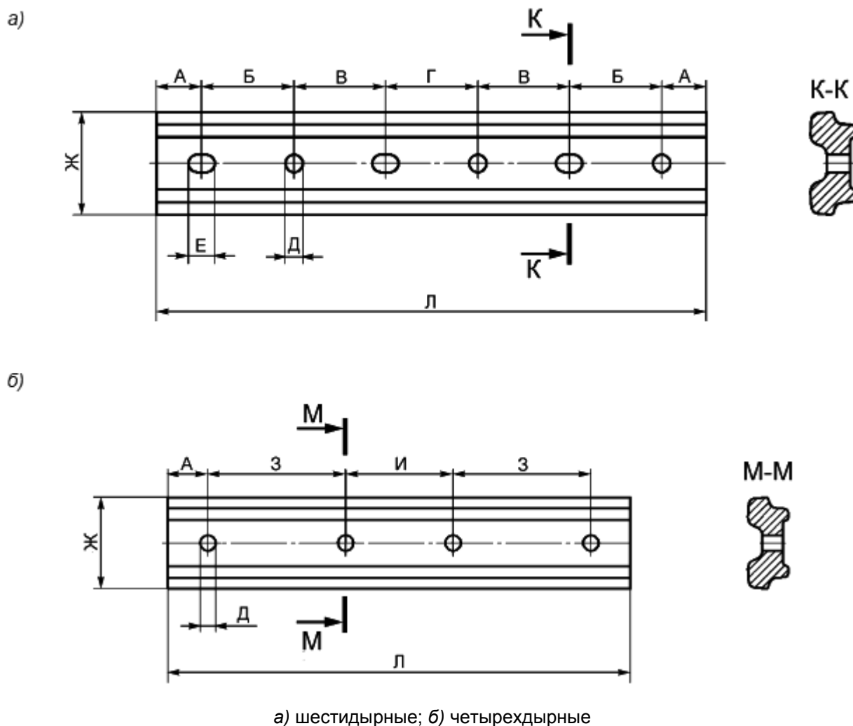
Рисунок А.1 - Двухголовые накладки для стыков железнодорожных рельсов Таблица А.1 - Размеры двухголовых накладок для стыков железнодорожных рельсов
