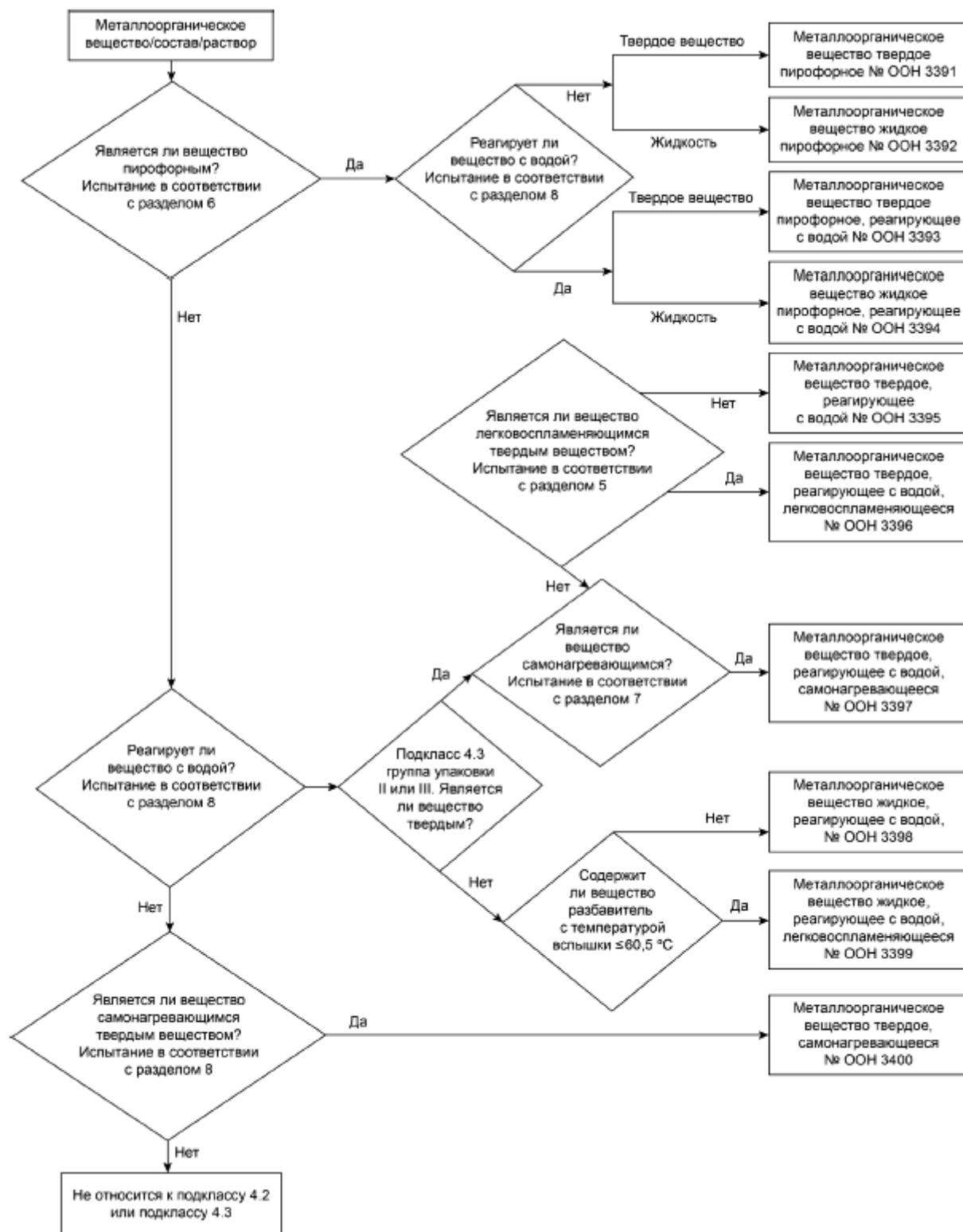
Рисунок Б.3 - Схема классификации металлоорганических веществ
