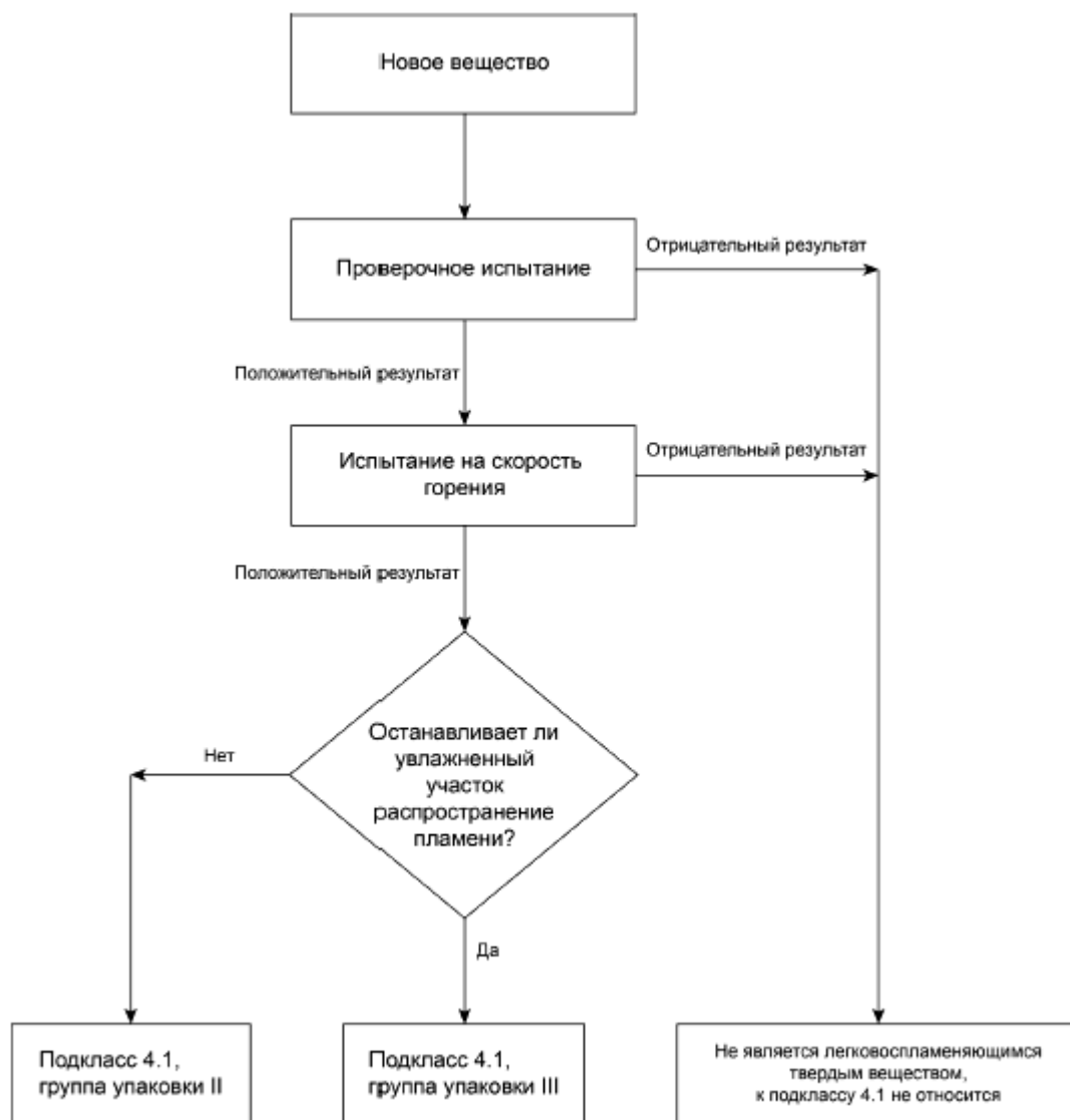
Рисунок Б.1 - Схема отнесения твердых веществ, способных легко воспламеняться (за исключением порошков металлов), к подклассу 4.1
