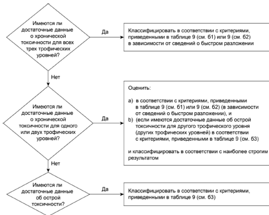
Рисунок Б.4 - Категории веществ, характеризующихся длительно действующей опасностью для водной среды
