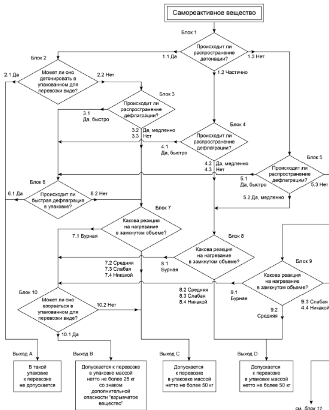
Рисунок Б.7 - Схема принятия решения относительно условий перевозки самореактивных веществ подкласса 4.1, лист 1 из 2
