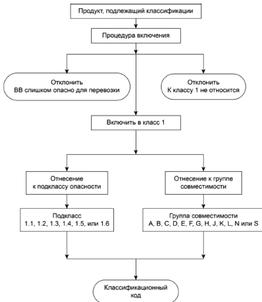
Рисунок Б.6 - Схема процедуры классификации вещества или изделия класса 1
