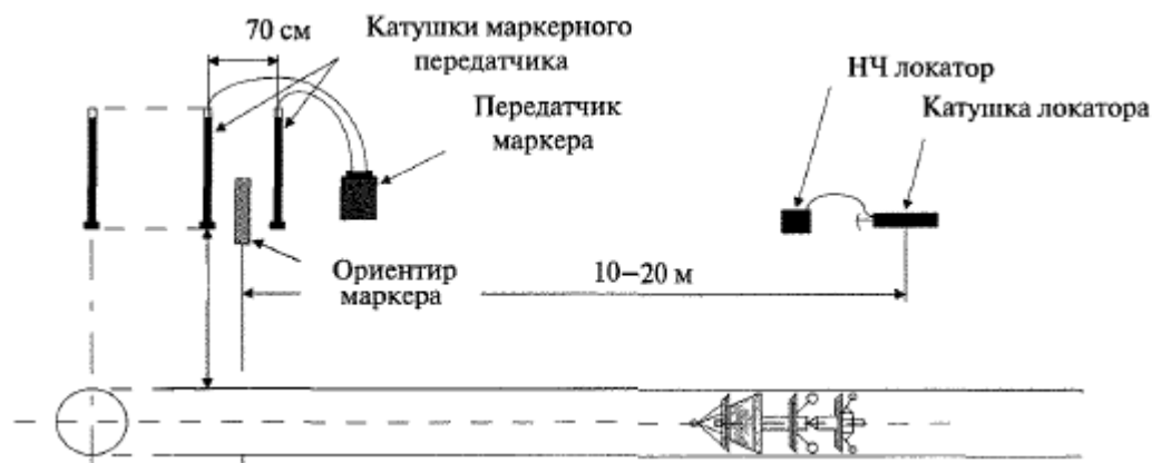
Рисунок 4. Размещение локатора и маркерного передатчика
