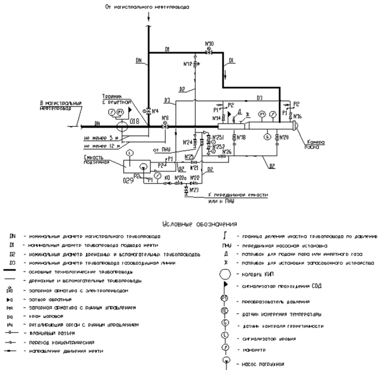
Рисунок 2. Технологическая схема узла пуска СОД на линейной части МТ
