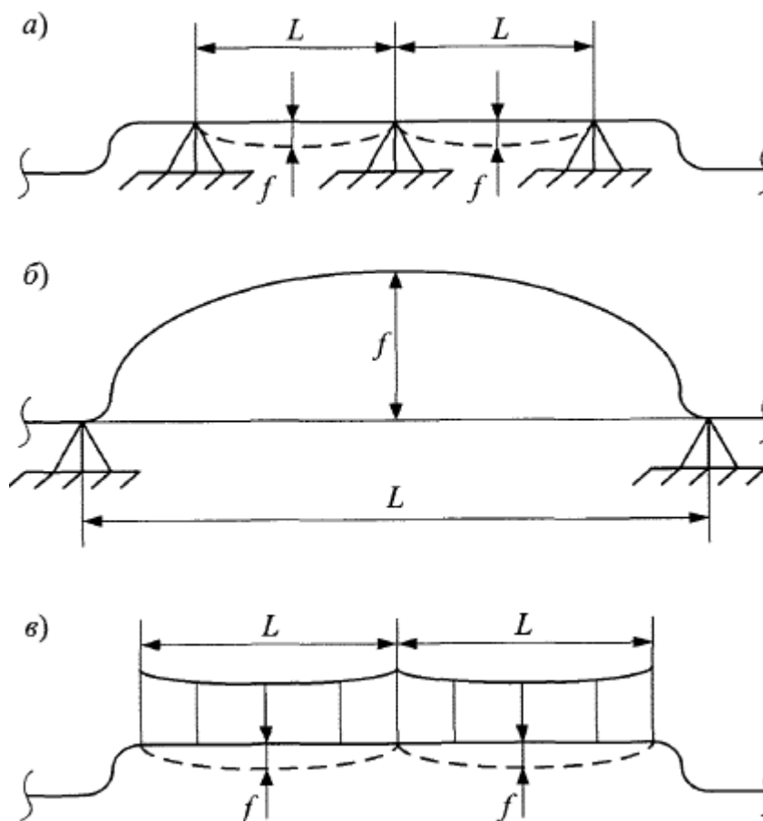
Рисунок 1. Схемы воздушных переходов и основные контролируемые геометрические параметры а) балочный переход; б) арочный переход; в) подвесной (вантовый) переход, L - длина пролета, f - стрела прогиба
