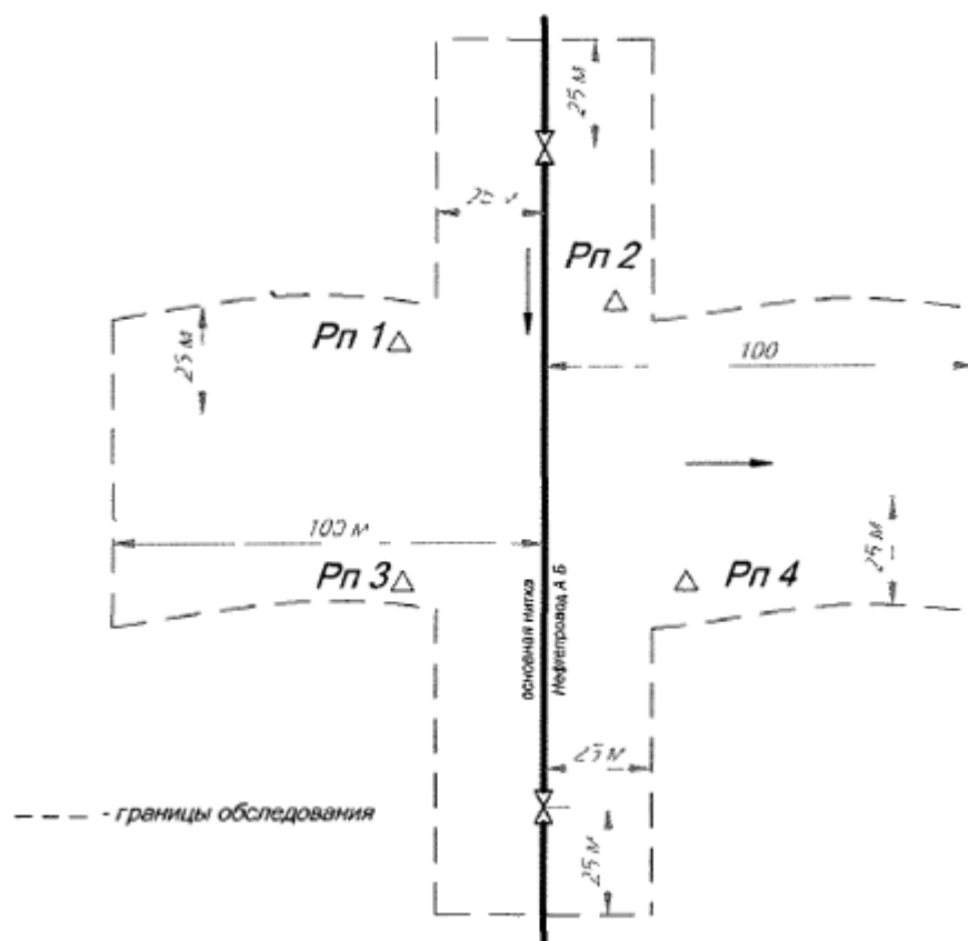
Рисунок 3. Границы обследования основной нитки одностороннего ППМТ, оборудованного запорной арматурой
