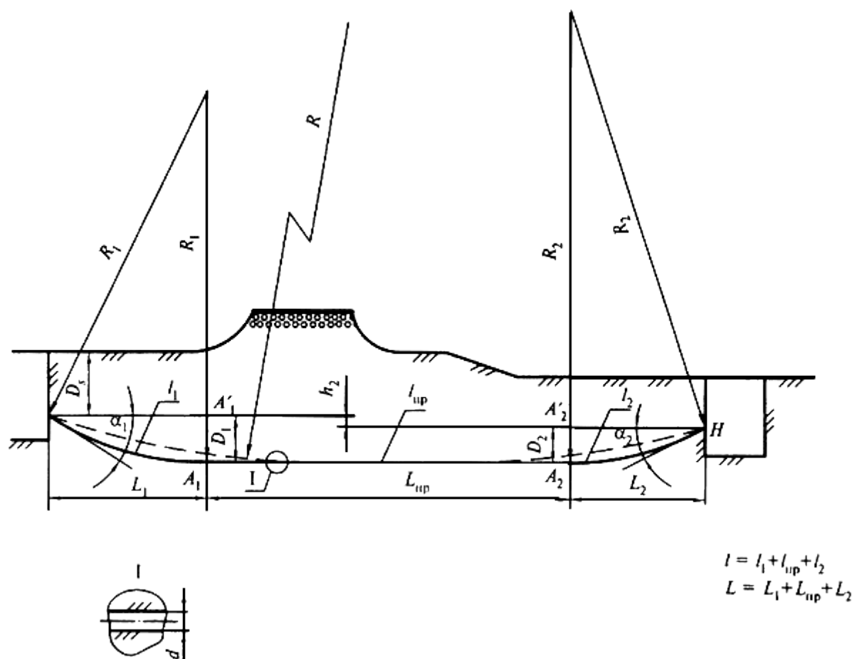
Рисунок Л.1 - Основные геометрические параметры трассы
