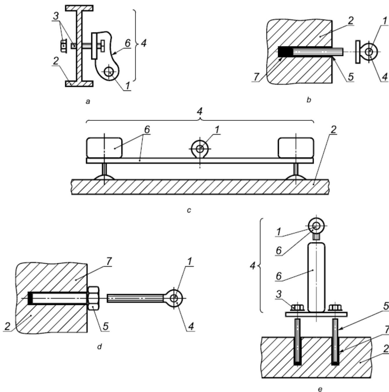
1 - анкерная точка; 2 - структура (не является частью анкерного устройства); 3 - элемент крепления; 4 - анкерное устройство; 5 - структурный анкер (не является частью анкерного устройства); 6 - элемент; 7 - постоянное крепление (например, склеивающая смола) Рисунок 1 - Примеры анкерных систем, которые включают в себя анкерное устройство
