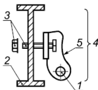
Рисунок 4 - Пример анкерного устройства типа А с элементом крепления
