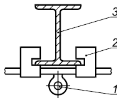
д – зажим на балку
