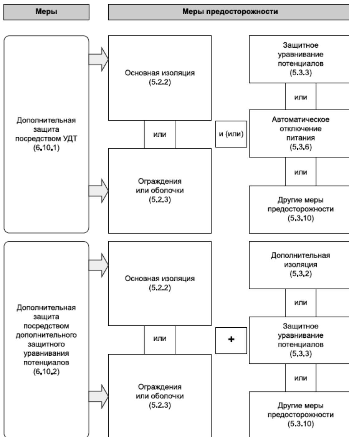
Рисунок А.3 - Дополнительная защита [в дополнение к основной защите и (или) защите при повреждении] Приложение В (справочное)
