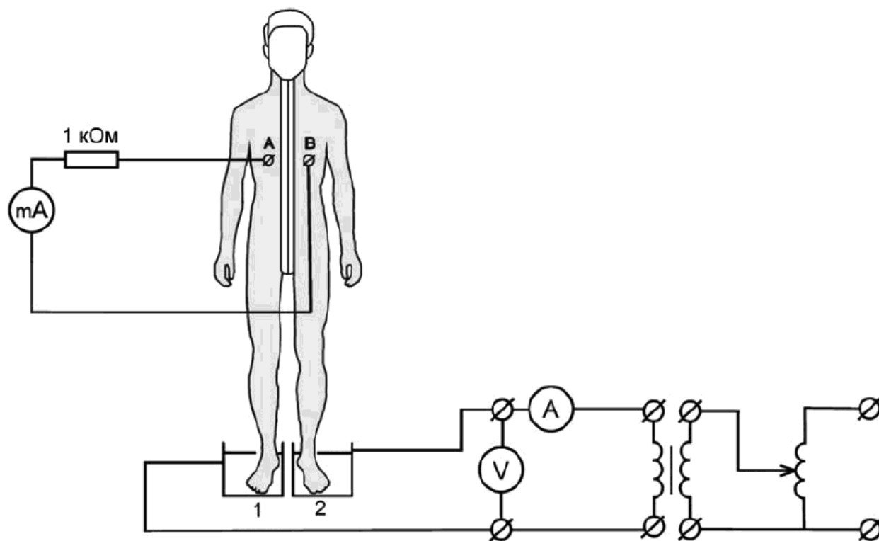
1, 2 - ванны
