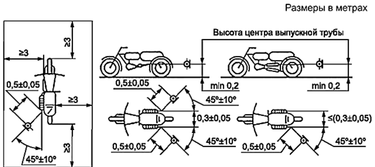
Рисунок К.2* - Расположение микрофона для измерения шума выпуска отработавших газов КТС категорий L
