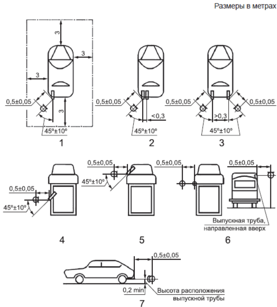
Рисунок К.1* - Расположение микрофона для измерения шума выпуска отработавших газов КТС категорий М и N
