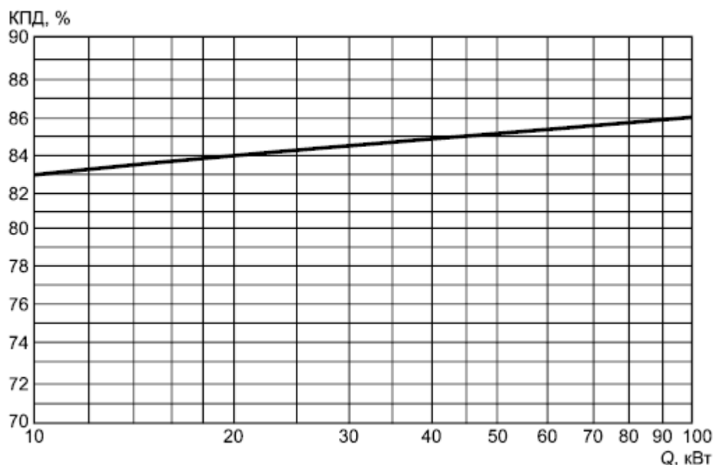
Рисунок 2 - График зависимости КПД котлов, оборудованных атмосферными горелками для сжигания газа, от теплопроизводительности
