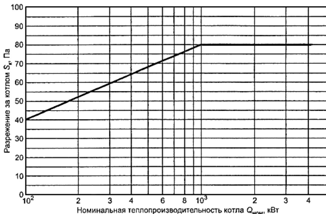
Рисунок 2 - Максимальное разрежение за котлом на естественной тяге
