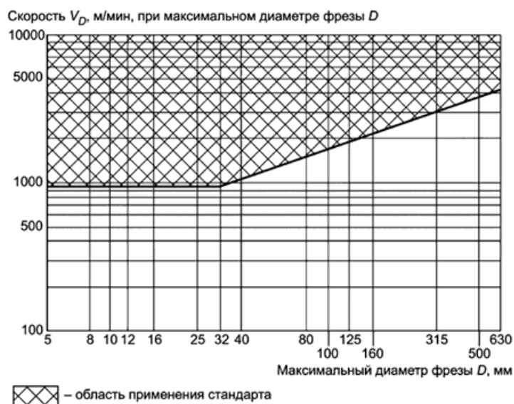
Рисунок 2 - Скорость V_D в зависимости от максимального диаметра фрезы D Пояснения к области применения приведены в приложении А.
