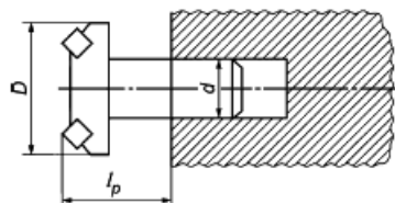
Рисунок 4 - Пример для сборной фрезы
