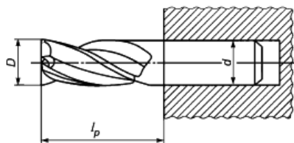
Рисунок 3 - Пример для цельной или составной фрезы
