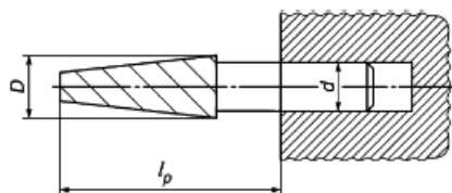
Рисунок 5 - Пример для цельной или составной конической фрезы
