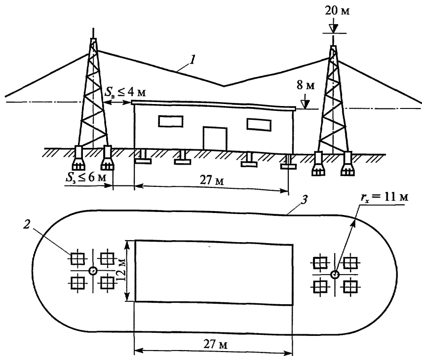
Рис. 3. Молниезащита здания I категории отдельно стоящим двойным стержневым молниеотводом ( \rho = 300 \text{ Ом} \cdot \text{м} , S_b \leq 4 \text{ м} , S_s \leq 6 \text{ м} ): 1 — граница зоны защиты; 2 — заземлители — подножки фундамента; 3 — зона защиты на отметке 8,0 м
