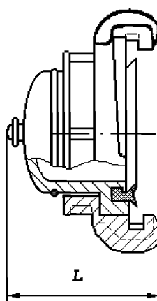
Рисунок 9 — Всасывающая головка-заглушка
