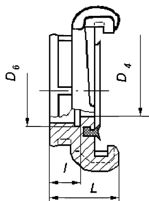
Рисунок 8 — Муфтовая всасывающая головка
