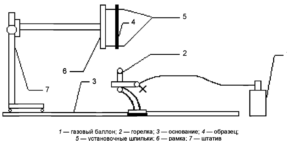
Рисунок 2 — Схема установки для испытания текстильных материалов на устойчивость к воздействию открытого пламени
