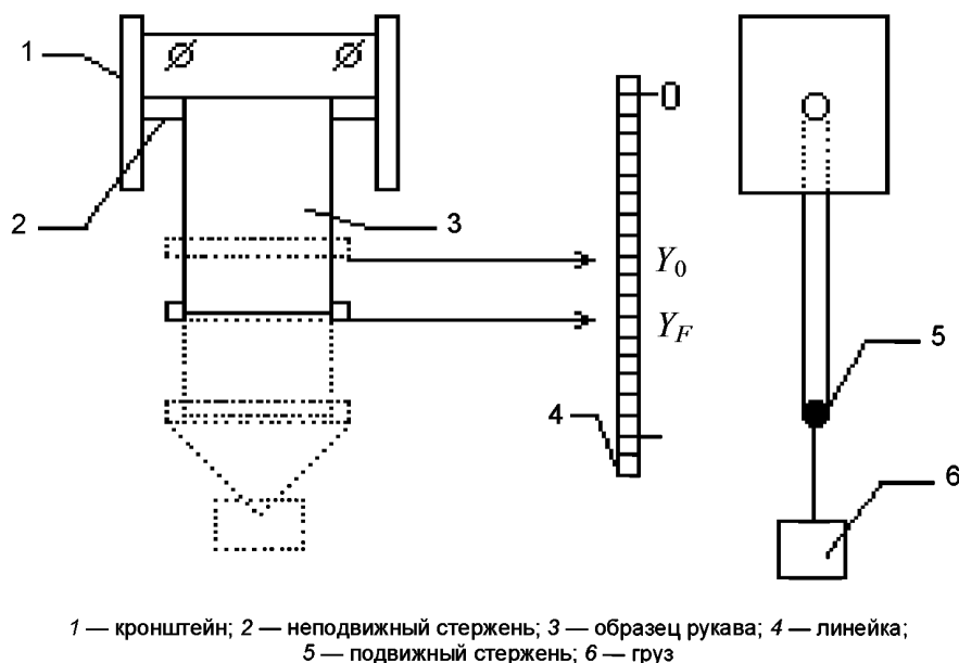
Рисунок 3 — Установка для определения растяжения образца эластичного рукава
