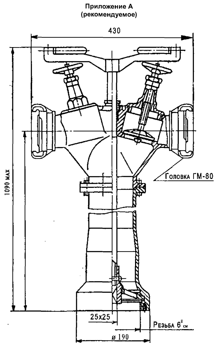
Рисунок А1 — Колонка пожарная
