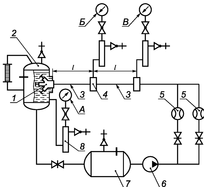
Рисунок Б.1 — Схема стэнда для проверки коэффициента гидравлического сопротивления
