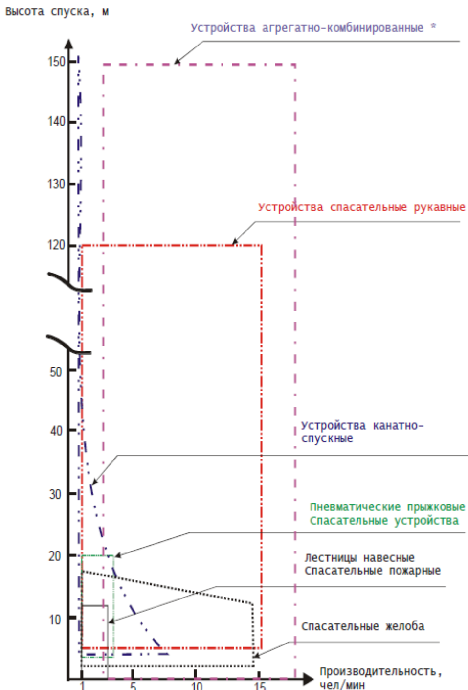
Рисунок 1 - Ориентировочная область применения устройств спасения с высоты различных типов.
