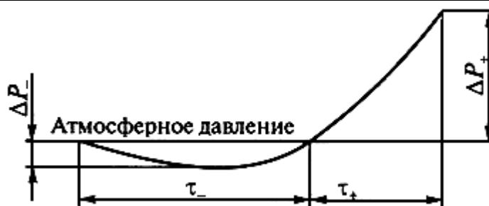
Рис.2. Характерный профиль ударной волны
