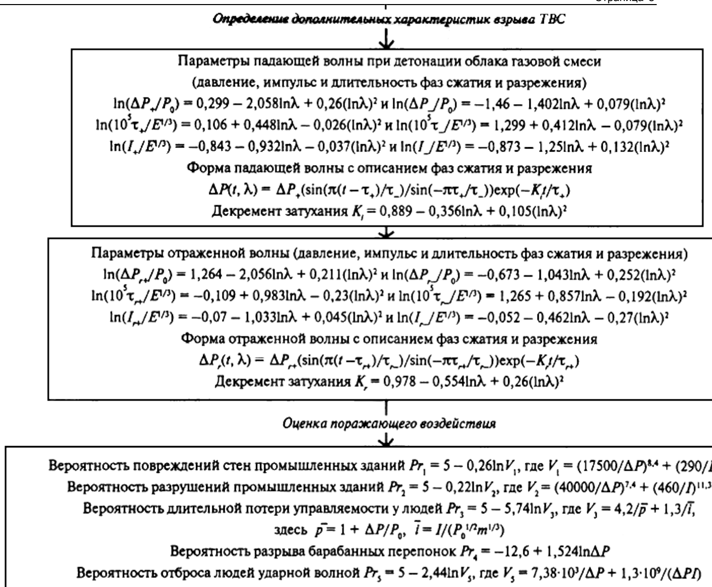
Рис.1. Алгоритм расчета последствий аварийных взрывов топливно-воздушных смесей 1.6. В приложении к Методике приведены примеры расчетов.
