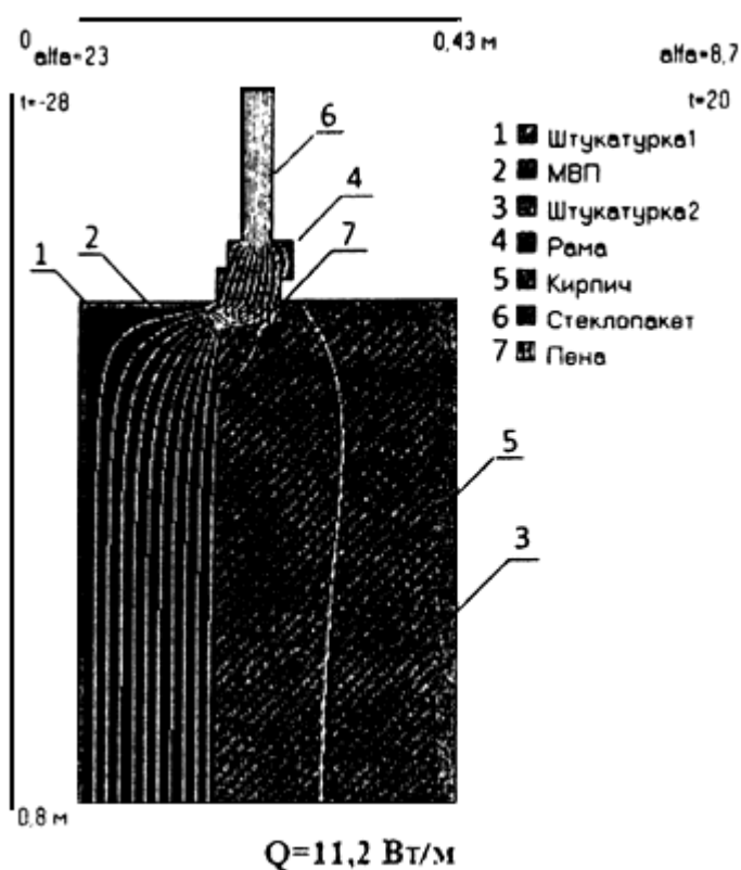
Рисунок Н.3 - Температурное поле узла конструкции, содержащего линейный элемент 2 Расчеты удельных характеристик других элементов проводятся аналогично и сведены в таблицу Н.2.
