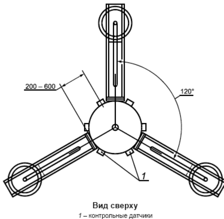
Рисунок 2 - Метод А: Схема расположения трех панелей с датчиками и двумя контрольными датчиками с каждой стороны
