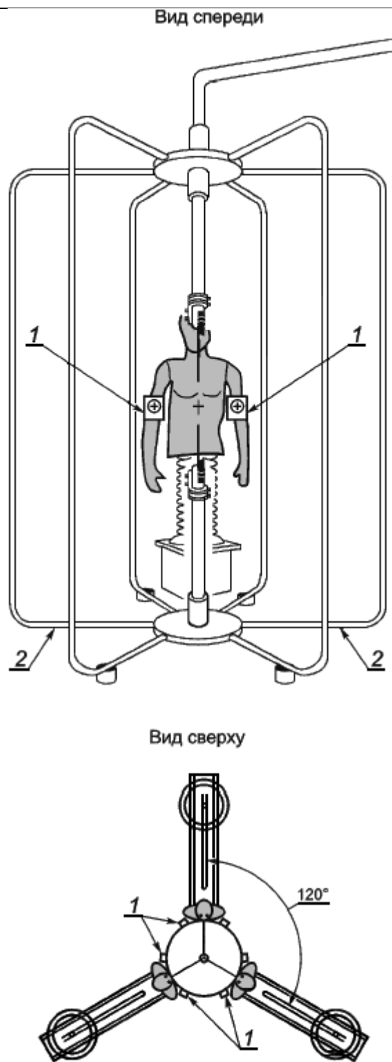
Рисунок 5 - Шина электропитания и электродуговые электроды относительно положения(ий) манекена(ов)
