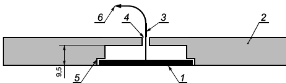
Рисунок 8 - Калориметр и детали термопары
