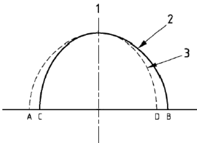
1 - испытательная ось; 2 - правый носок; 3 - левый носок
