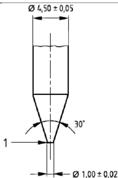
1 - усеченный наконечник
