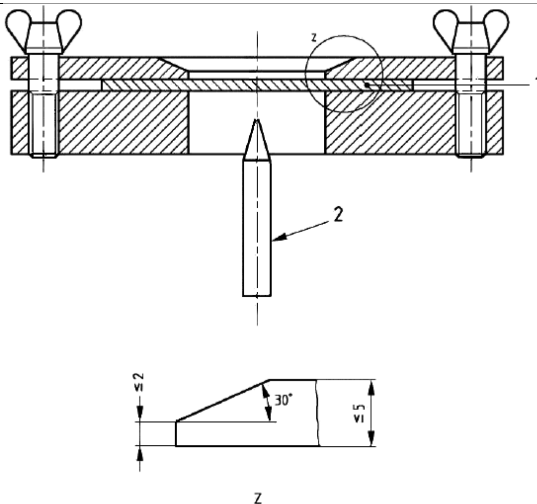
1 - испытуемый образец; 2 - испытательный гвоздь
