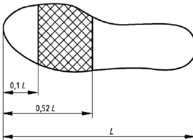
L - общая длина металлической стельки
