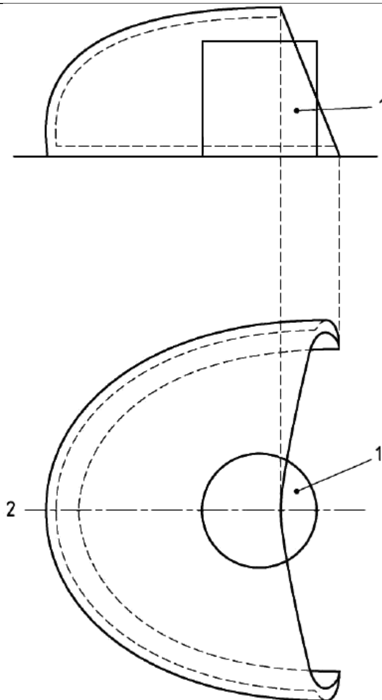
1 - цилиндр из глины; 2 - испытательная ось
