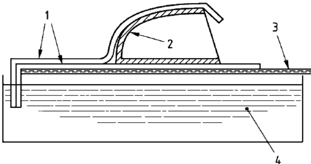
Рисунок 8 - Схема определения коррозии на металлических носках
