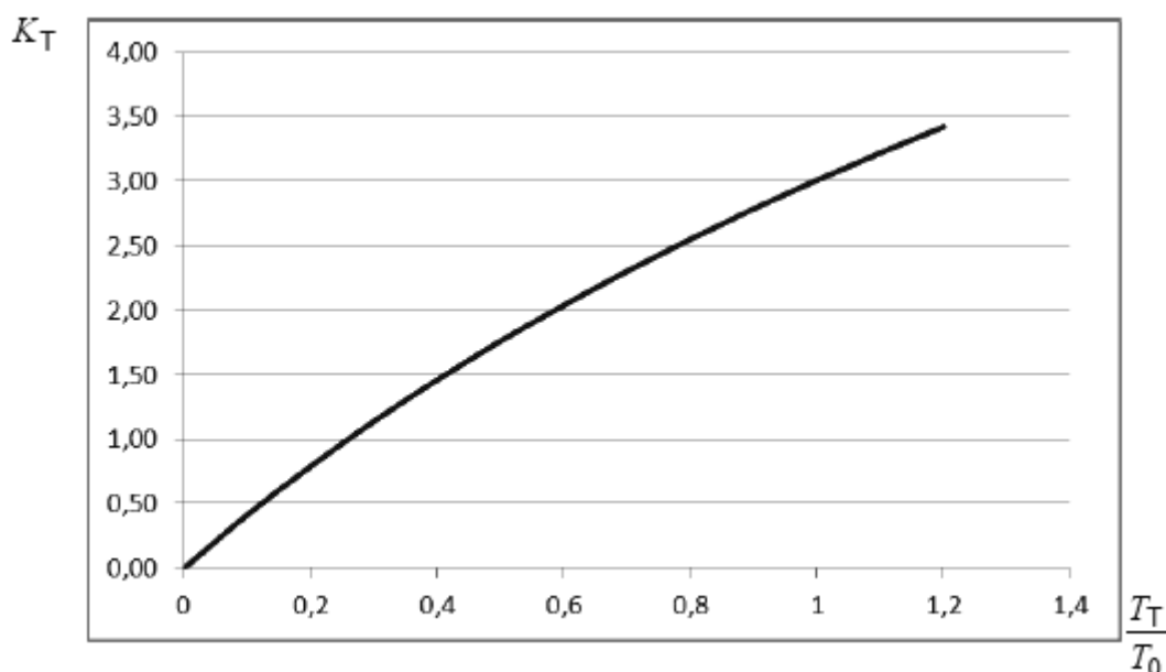
Рисунок А.1 - Зависимость K_T , дБ, от T_T / T_0
